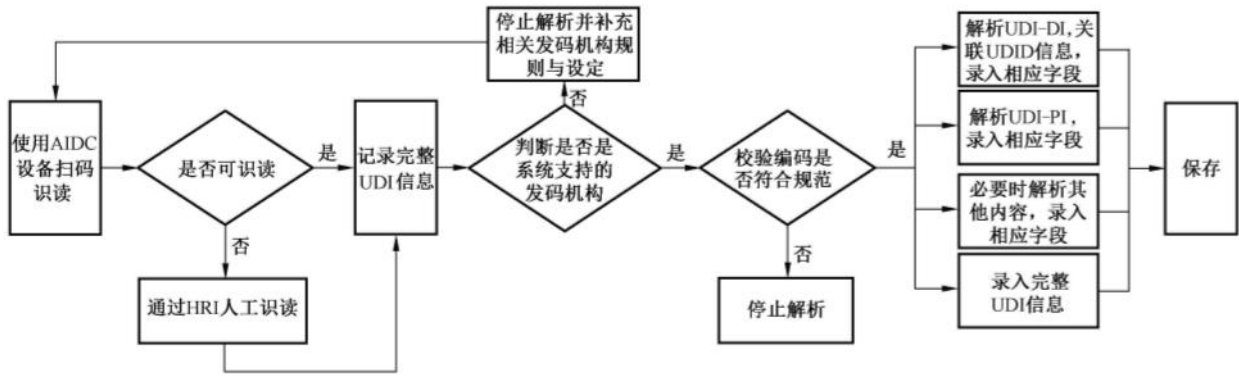
图 5 1 种在信息系统中记录 UDI 和相关信息的参考流程
