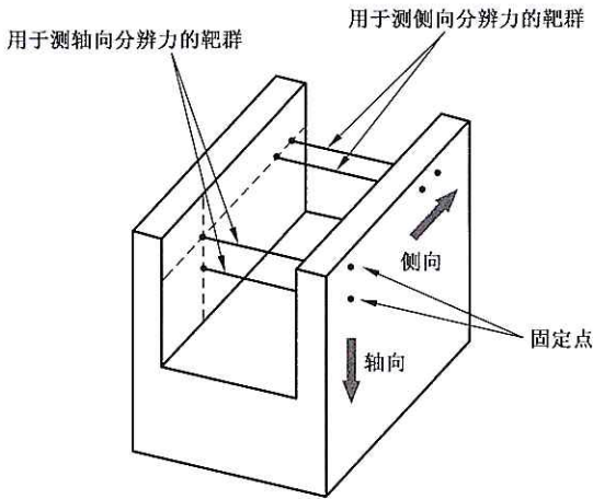
图 A.1 分辨力测量用弦线试件
