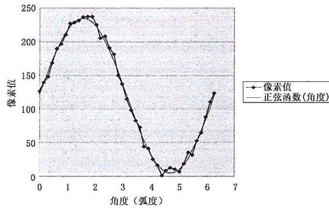
图 C.4 根据角度情况的数字码值
