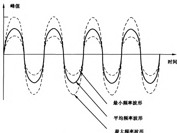
图 2 模拟多普勒信号频率的最小、平均和最大频率的正弦变化
