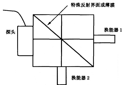
b) 探头与测试件换能器之间的另一种耦合方式
