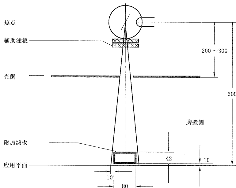
图 6 应用辐射条件 RQB-M 的测量布置
