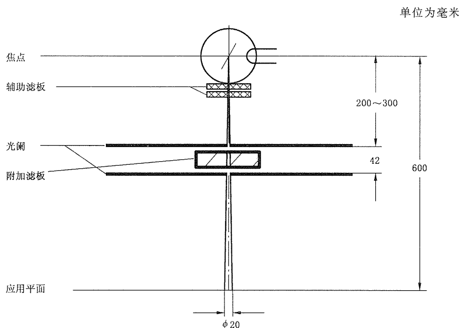
图 5 应用辐射条件 RQN-M 的测量布置
