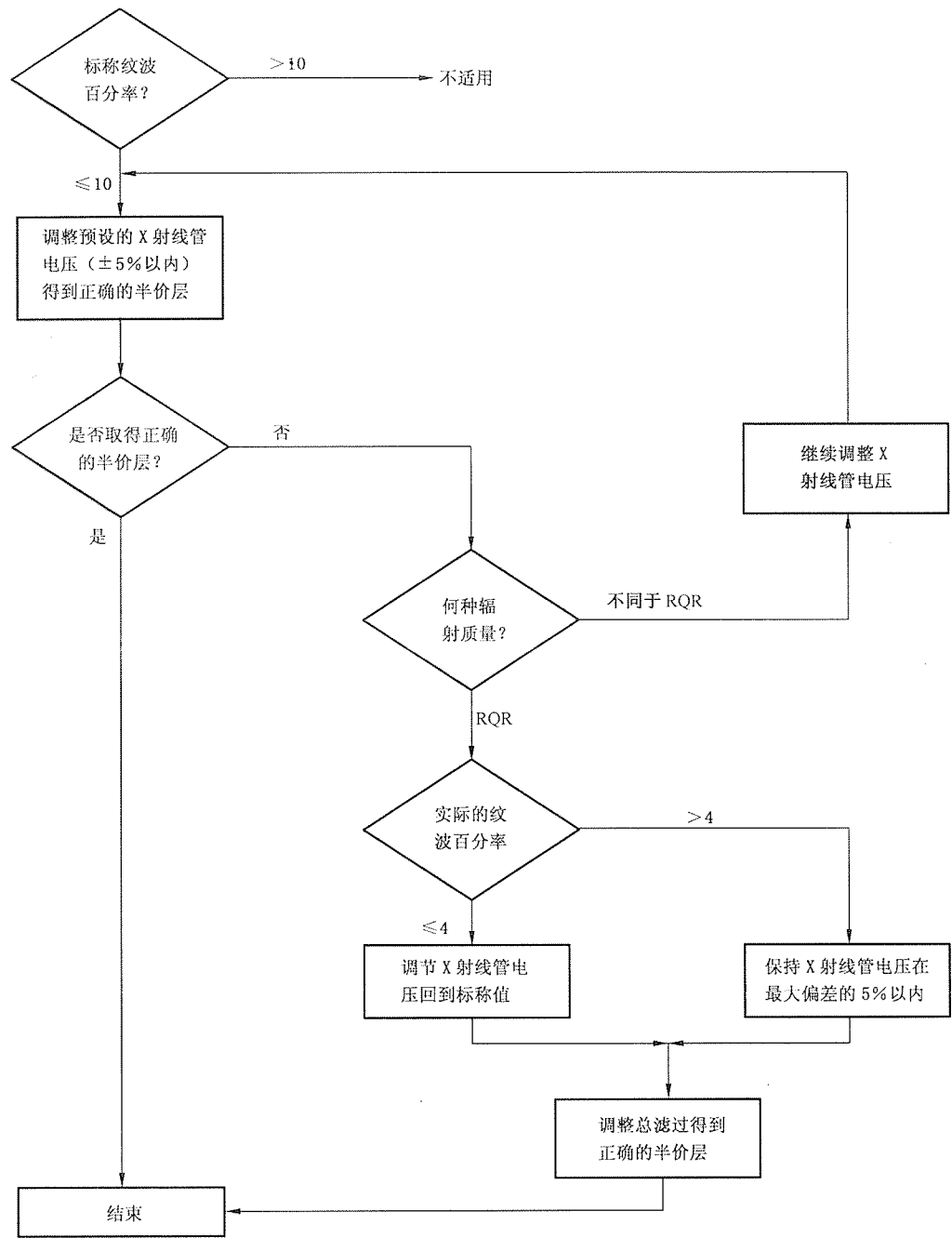
图7 建立标准辐射条件的调整程序
