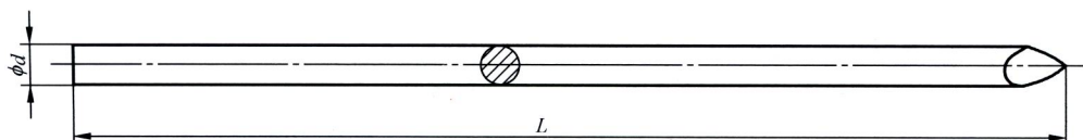
图 1 克氏针的主要尺寸
