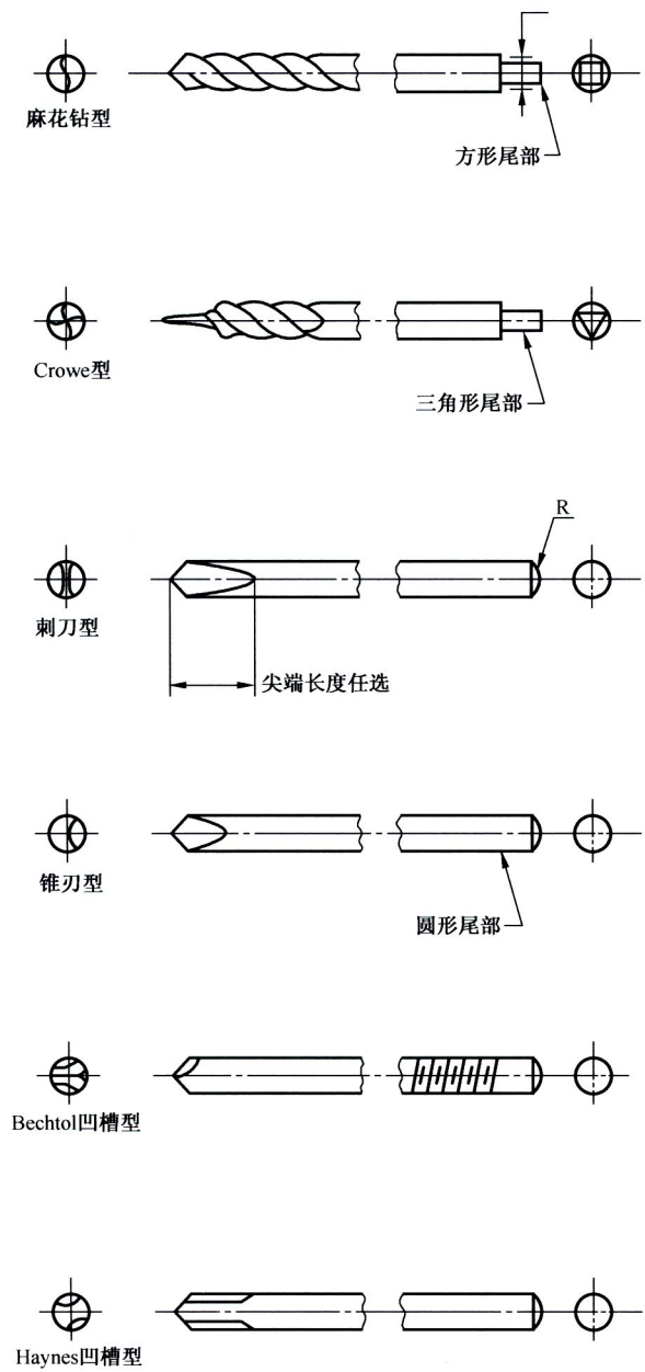
图 A.1 尖端和钝端
