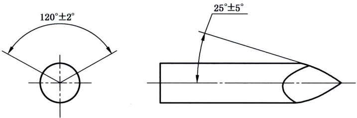
图 2 A 型:锥刃形尖端
