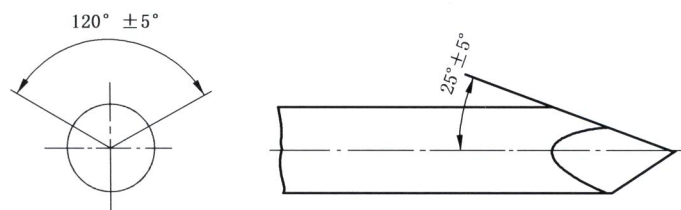
图2 斯氏针的推荐尖端
