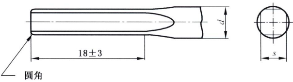
图 4 B 型:方形端部
