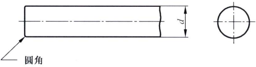
图 3 A 型:圆形端部
