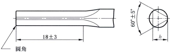
图 5 C 型:三角形端部
