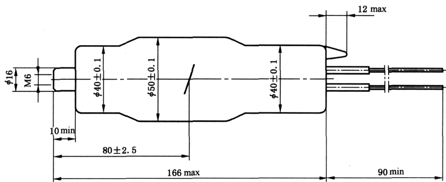
图 A.1 外形图
