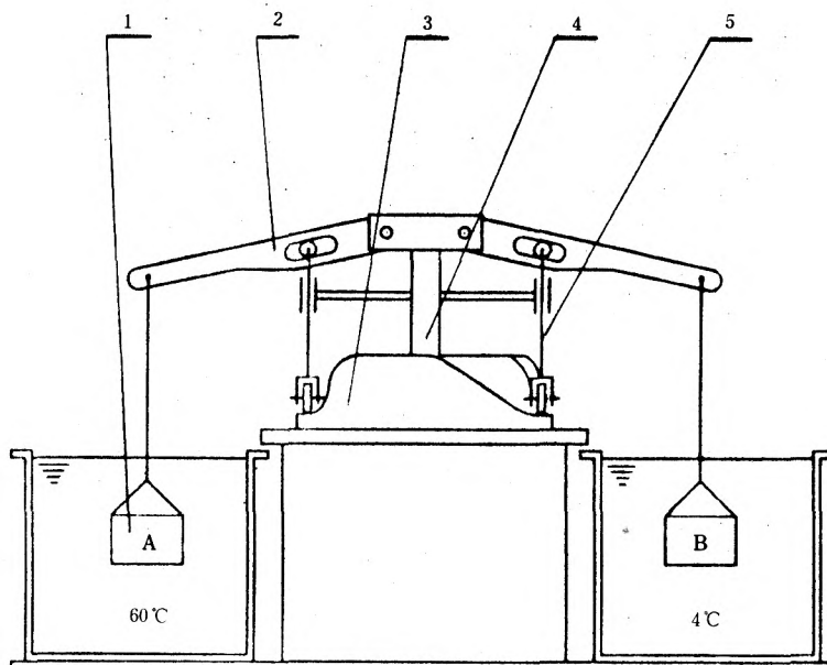
图 2 高低温交换装置工作部分
