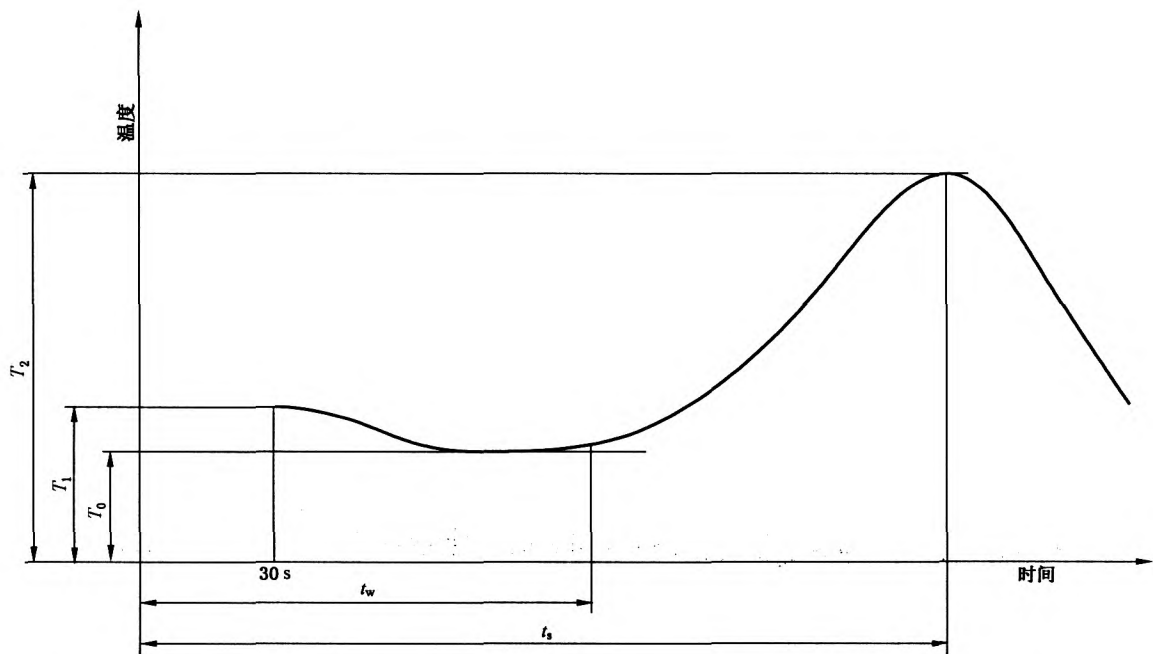
注：典型的记录曲线表明热电偶刚插入样品内的温度 T_1 ，插入后温度轻微下降 T_0 ，温度峰值 T_2 。温度开始上升的时间 t_w ，表示固化反应开始，也即工作时间的结束。温度峰值的时间 t_s ，表示固化时间。 图 2 典型的记录曲线显示测量工作时间及固化时间时温度随时间的变化
