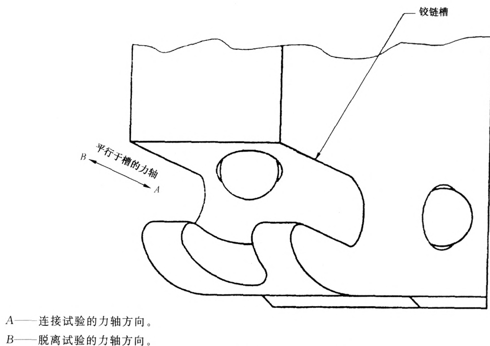
图 3 连接和脱离试验的力轴(见 3.5)
