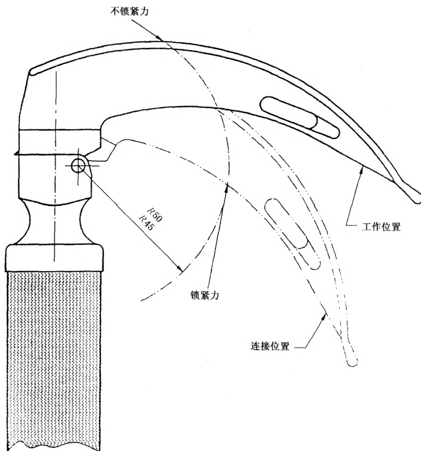
图 4 锁定接头试验的转矩应用(见 3.7.1 和 3.7.2)
