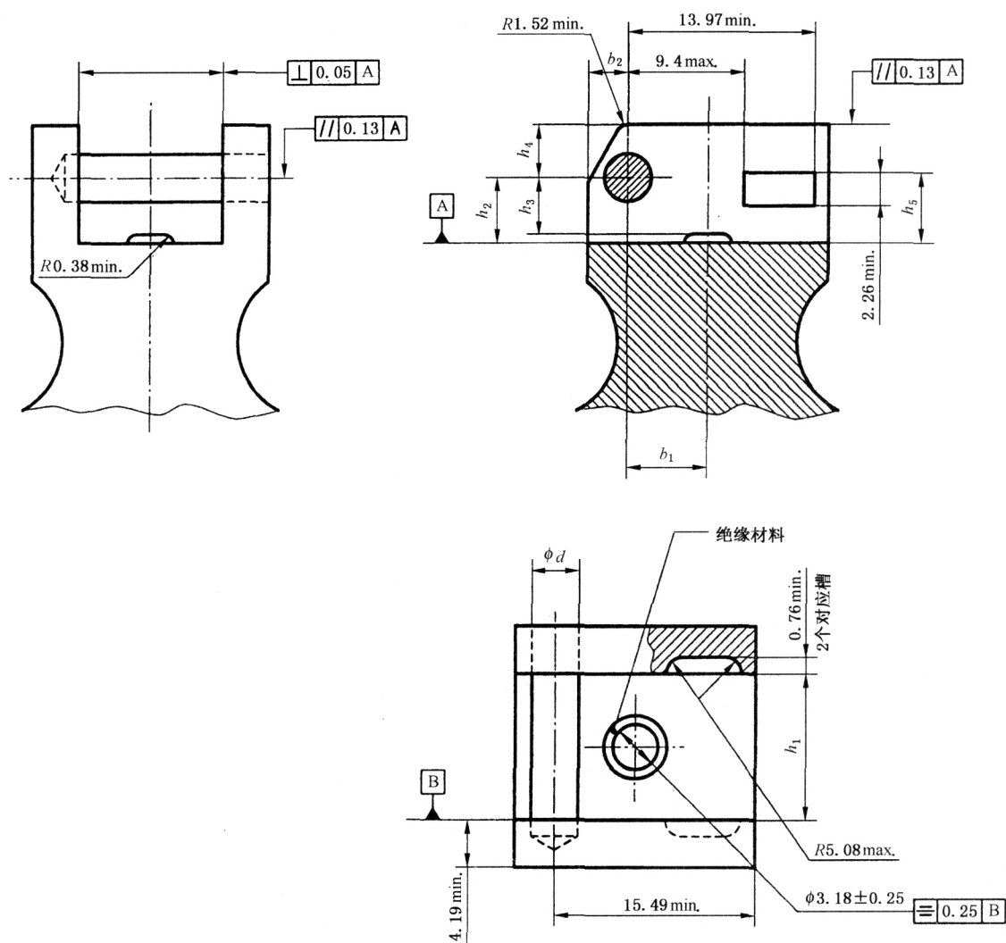
图 A.1 试验手柄接头
