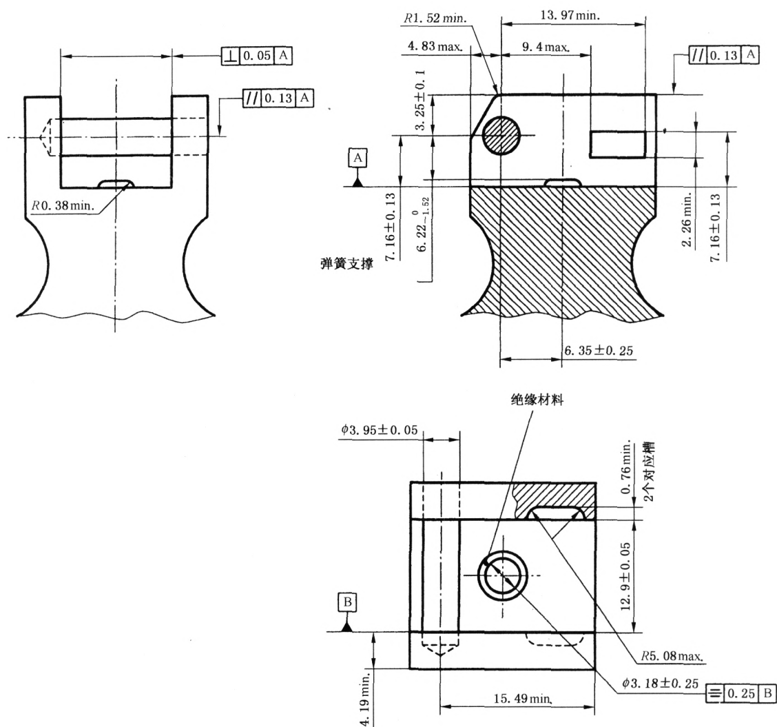
图 1 手柄接头
