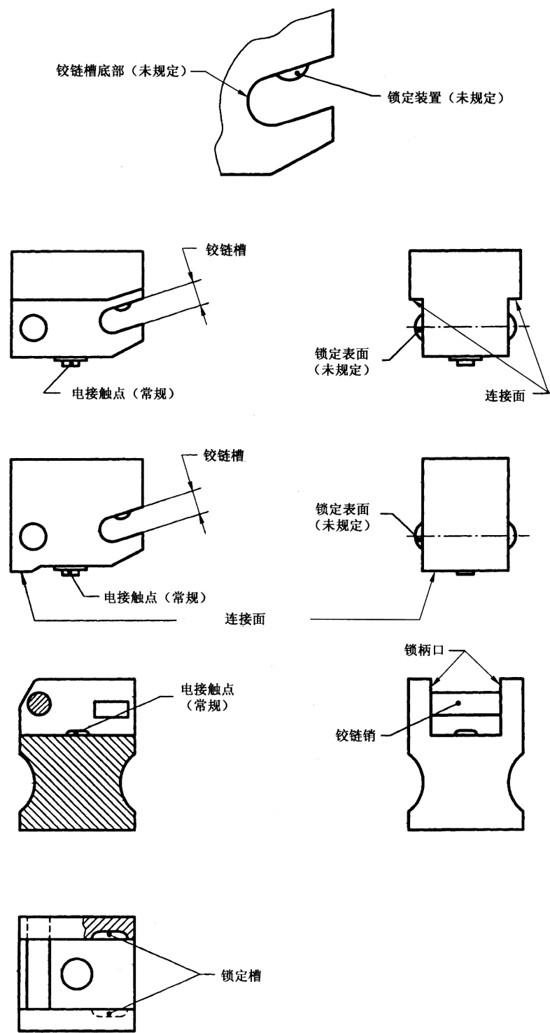
图 2 典型的窥视片接头型式
