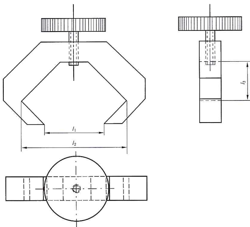
图3 三角形截面槽伸长仪 A—A 截面图
