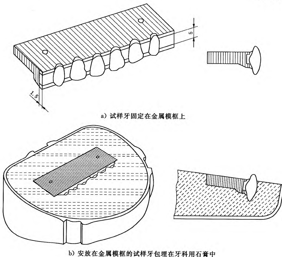
图 3 粘接试验用的装置和模具
