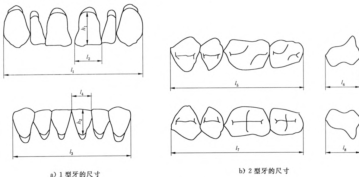
图 1 尺寸的测量
