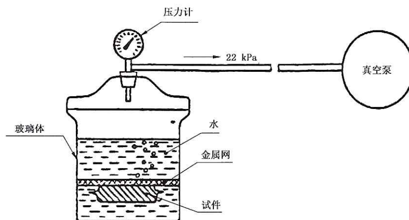
图 2 密封性测试装置
