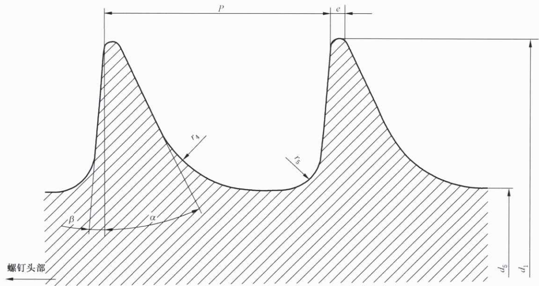
图 4 深螺纹(HB 型)
