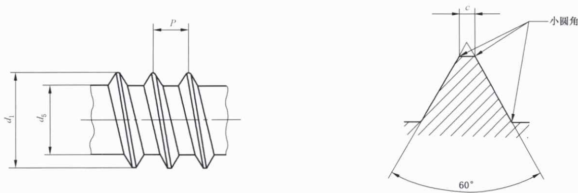
图 7 HC 型接骨螺钉螺纹
