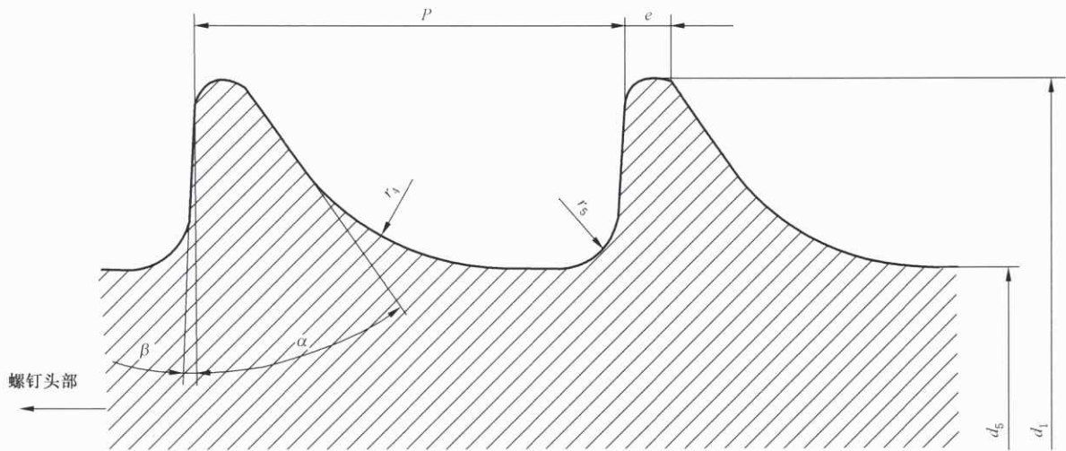
图 2 浅螺纹(HA 型)
