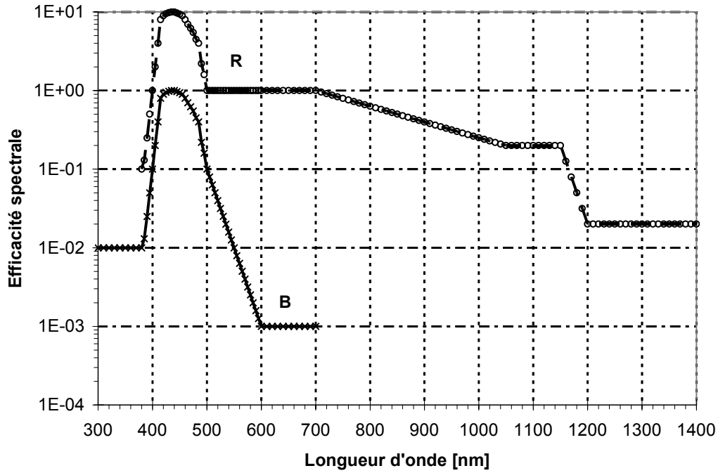
Figure 4.2 Fonctions de pondération spectrale pour les risques rétinien: B(\lambda) et R(\lambda) .
