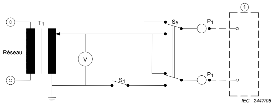
Figure F.1 – Circuit d'alimentation de mesure avec un côté du RÉSEAU D'ALIMENTATION approximativement au potentiel de terre (voir 8.7.4.2)
