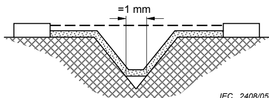
Figure 24 – LIGNE DE FUIITE et DISTANCE DANS L'AIR – Exemple 2
