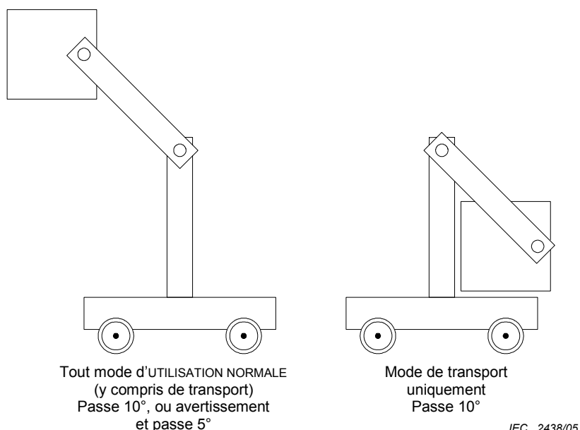
Figure A.16 – Conditions de l'essai d'instabilité
