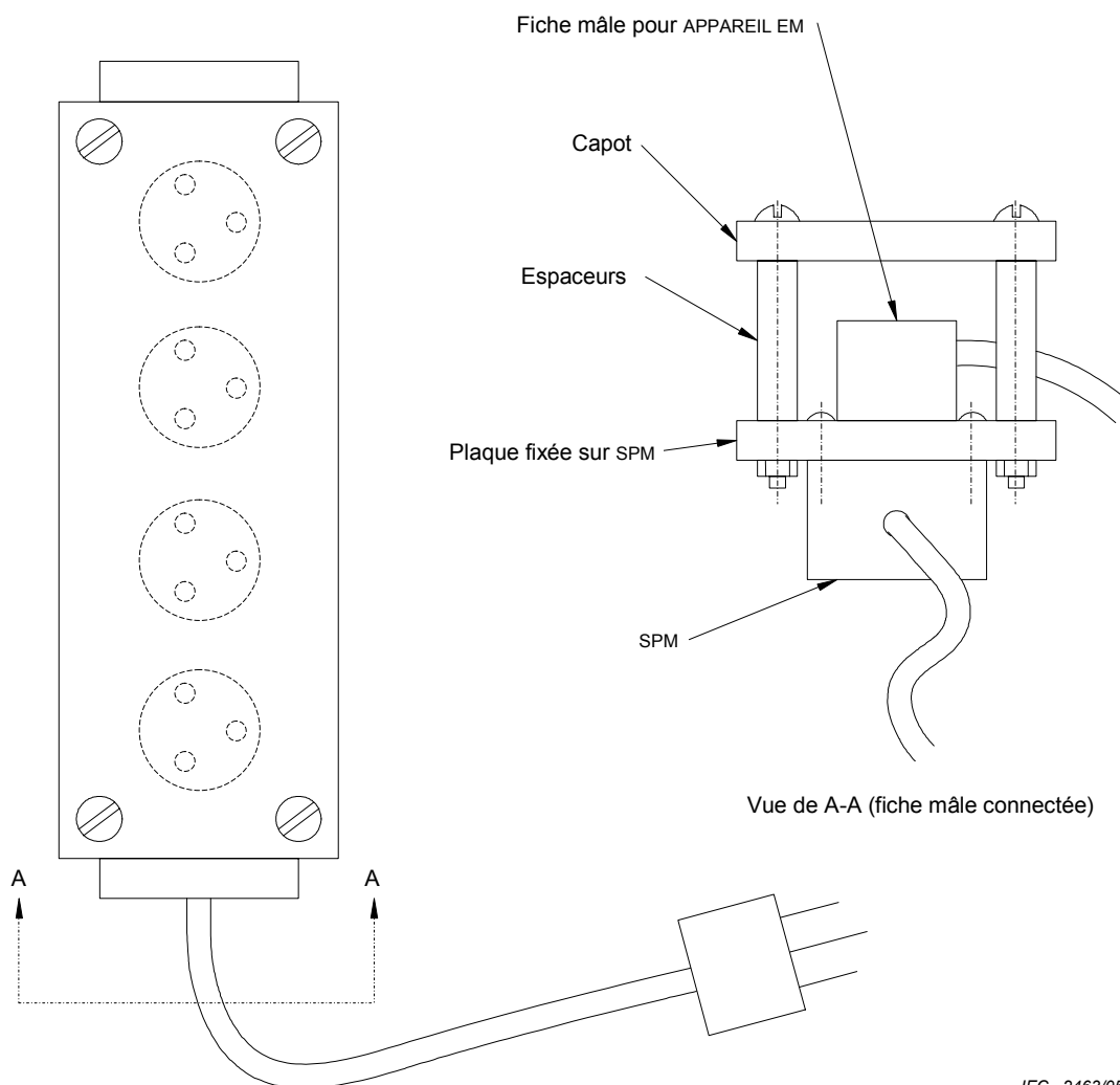
Figure I.1 – Exemple de construction de SOCLE DE PRISES MULTIPLES (SPM) (accessible uniquement à l'aide d'un outil)
