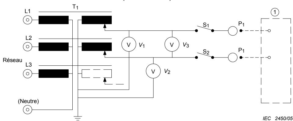
Figure F.3 – Circuit d'alimentation de mesure pour les APPAREILS EM polyphasés spécifiés pour connexion à un RÉSEAU D'ALIMENTATION polyphasé (voir 8.7.4.2)
