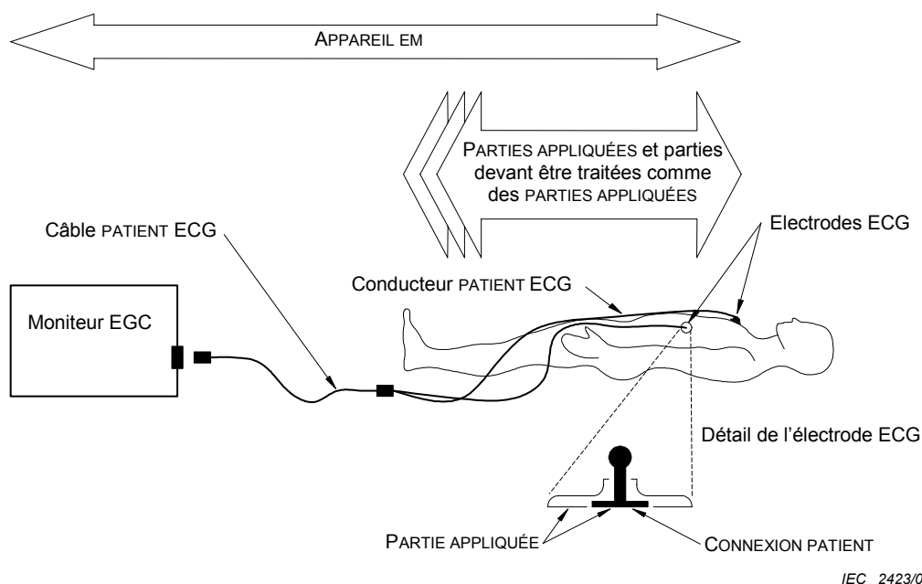
Figure A.1 – Identification de l'APPAREIL EM, des PARTIES APPLIQUÉES et des CONNEXIONS PATIENT dans un moniteur d'électrocardiogramme
