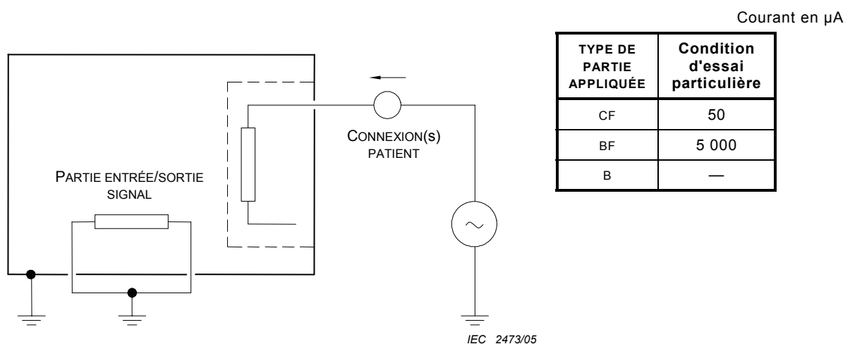
Figure K.1 – APPAREIL EM avec ENVELOPPE en matière isolante (Figure 15 simplifiée) (voir 8.7.4.7 a))
