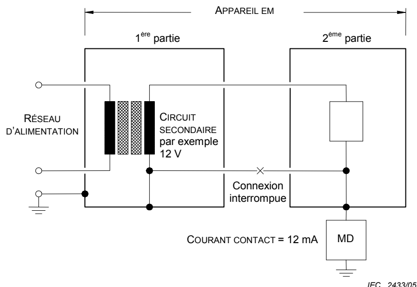
Figure A.11 – Interruption d'un conducteur d'alimentation entre des parties de l'APPAREIL EM dans des ENVELOPPES séparées
