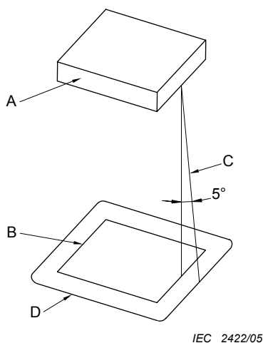
Figure 38 – Déflecteur (voir 11.3)
