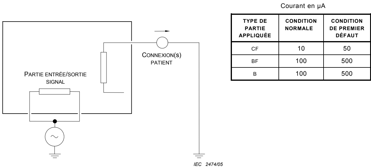
Exemple de circuit d'alimentation de mesure de la Figure F.1
