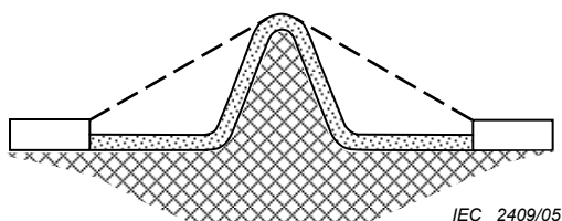
Figure 26 – LIGNE DE FUIITE et DISTANCE DANS L'AIR – Exemple 4
