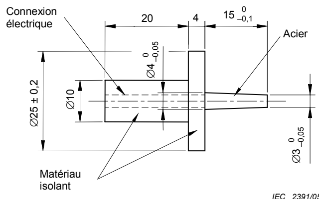
Figure 8 – Broche d'essai (voir 8.4.2 d) )
