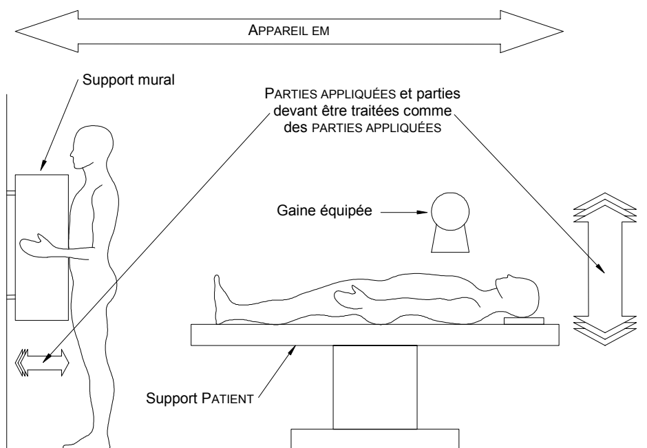
Figure A.5 – Identification des PARTIES APPLIQUÉES et des CONNEXIONS PATIENT dans un SYSTÈME EM À RAYONS X
