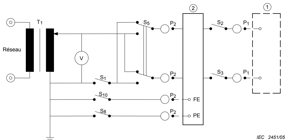
Figure F.5 – Circuit d'alimentation de mesure pour les APPAREILS EM ayant une unité d'alimentation séparée ou destiné à recevoir sa puissance d'un autre appareil du SYSTÈME EM (voir 8.7.4.2)
