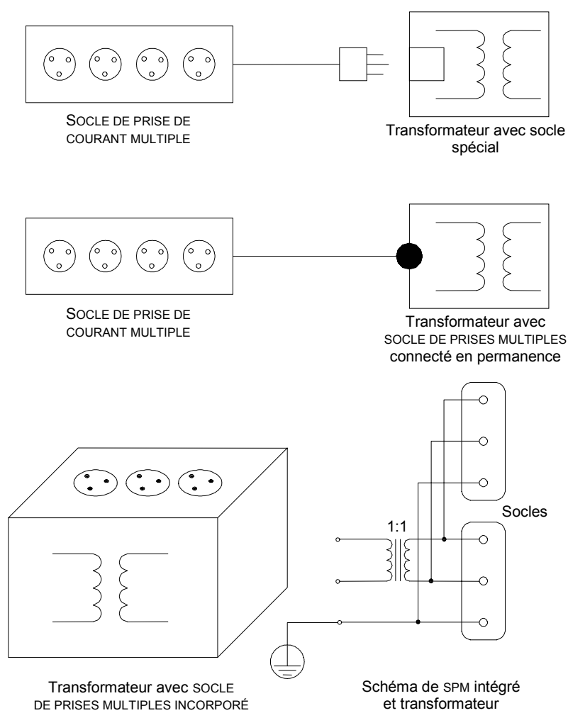
Figure I.2 – Exemples d'application de SOCLES DE PRISES MULTIPLES (SPM)
