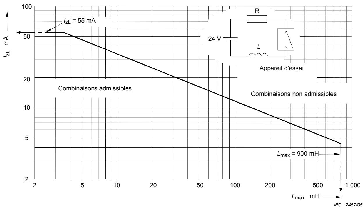
Figure G.6 – Courant maximal admissible I_{zL} en fonction de l'inductance L_{max} mesurée dans un circuit inductif avec le mélange le plus facilement inflammable de vapeur d'éther et d'oxygène
