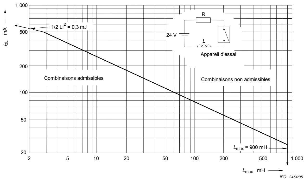
Figure G.3 – Courant maximal admissible I_{ZL} en fonction de l'inductance L_{\max} mesurée dans un circuit inductif avec le mélange le plus facilement inflammable de vapeur d'éther et d'air
