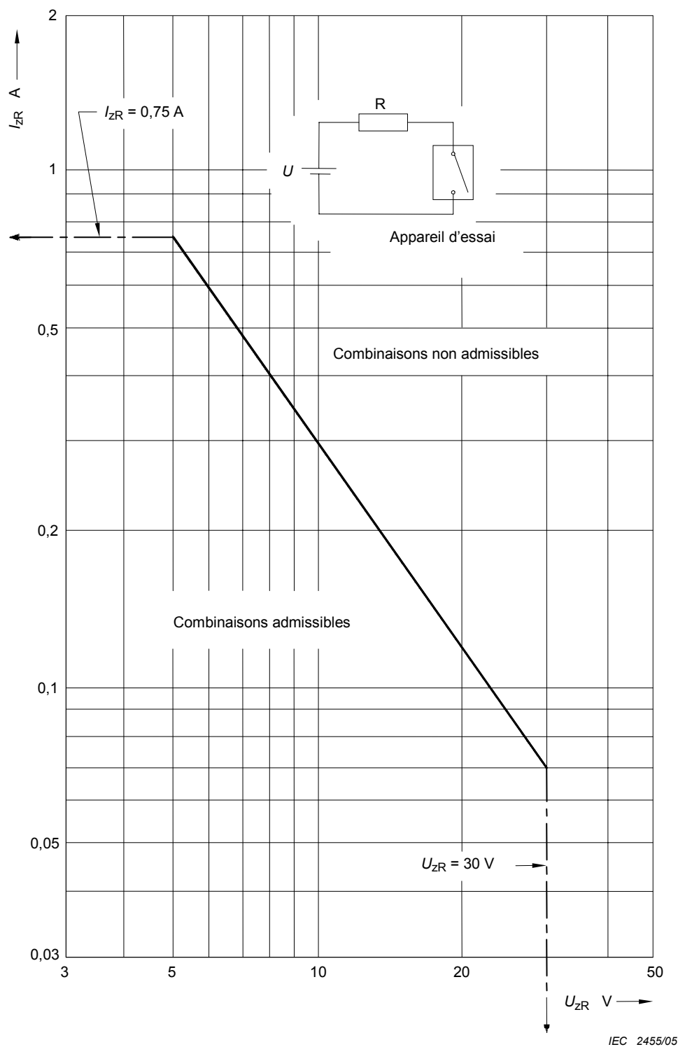
Figure G.4 – Courant maximal admissible I_{ZR} en fonction de la tension maximale admissible U_{ZR} mesuré dans un circuit purement résistif avec le mélange le plus facilement inflammable de vapeur d'éther et d'oxygène
