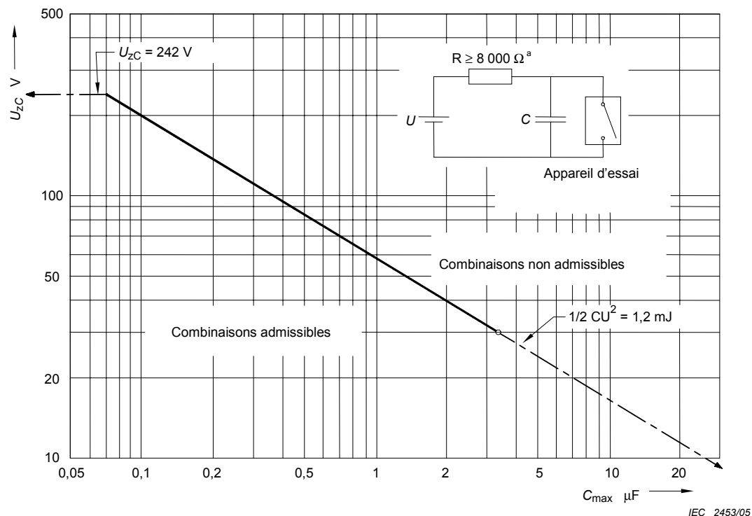
Figure G.2 – Tension maximale admissible U_{ZC} en fonction de la capacité C_{\max} mesurée dans un circuit capacitif avec le mélange le plus facilement inflammable de vapeur d'éther et d'air
