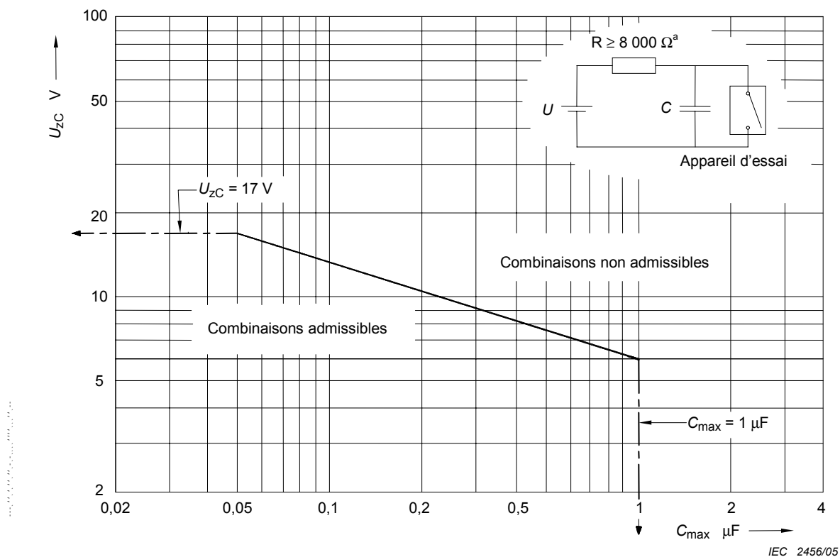
Figure G.5 – Tension maximale admissible U_{zC} en fonction de la capacité C_{max} mesurée dans un circuit capacitif avec le mélange le plus facilement inflammable de vapeur d'éther et d'oxygène
