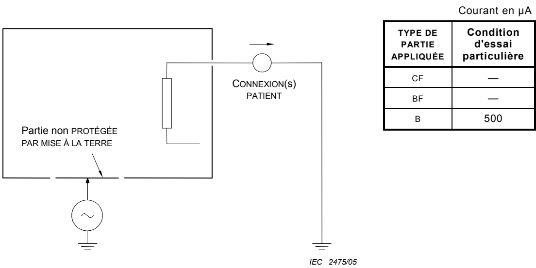
Figure K.3 – APPAREIL EM avec une PARTIE APPLIQUÉE et une PARTIE E/S DE SIGNAL (Figure 17 simplifiée) (voir 8.7.4.7 c))
