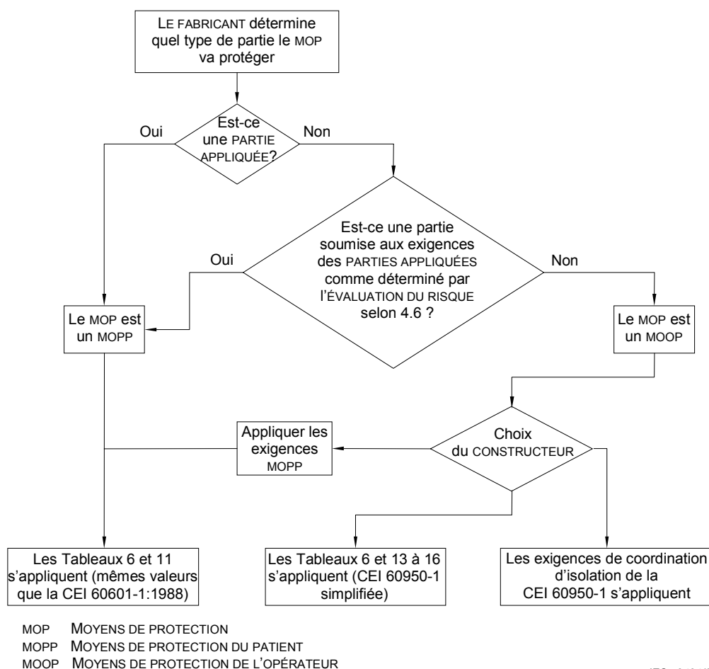
Figure A.12 – Identification des MOYENS DE PROTECTION DU PATIENT et des MOYENS DE PROTECTION DE L'OPÉRATEUR
