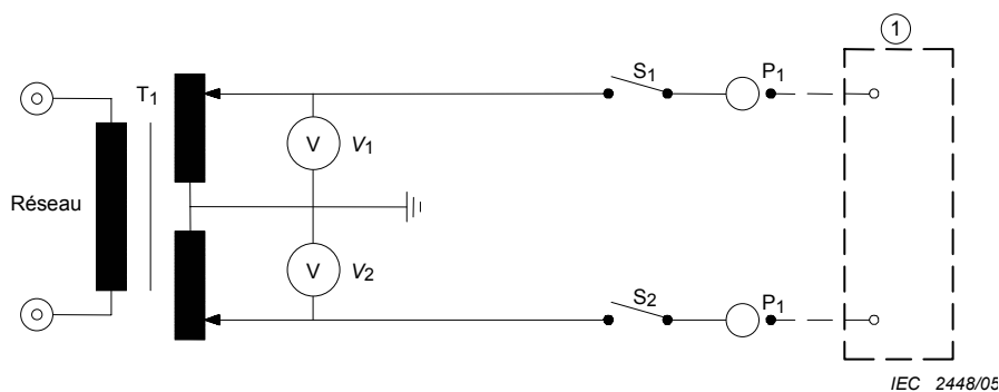
Figure F.2 – Circuit d'alimentation de mesure avec RÉSEAU D'ALIMENTATION approximativement symétrique au potentiel de terre (voir 8.7.4.2)
