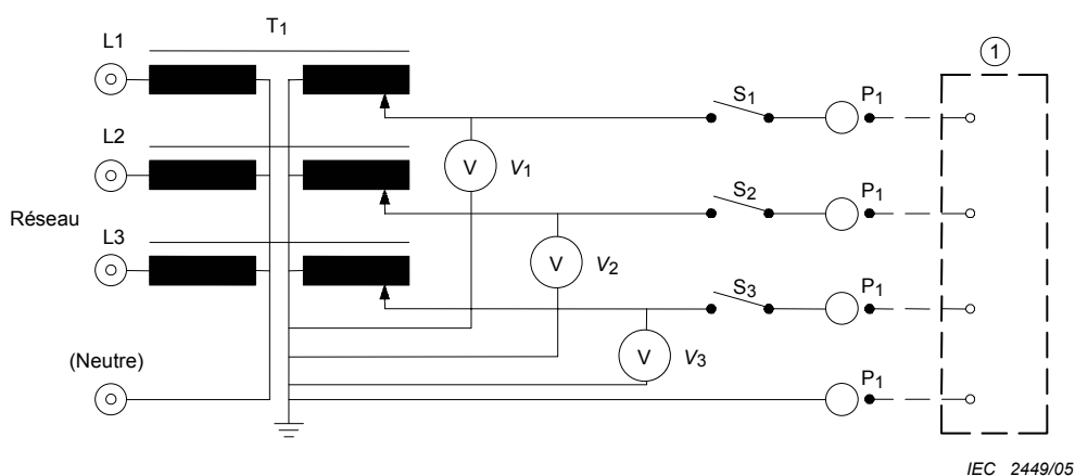
Figure F.3 – Circuit d'alimentation de mesure pour les APPAREILS EM polyphasés spécifiés pour connexion à un RÉSEAU D'ALIMENTATION polyphasé (voir 8.7.4.2)
