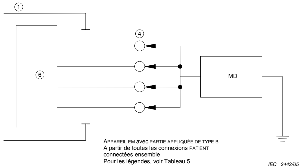
Figure E.1 – PARTIE APPLIQUÉE DE TYPE B
