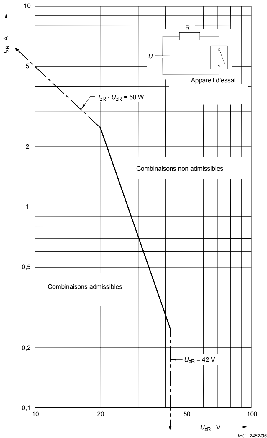
Figure G.1 – Courant maximal admissible I_{ZR} en fonction de la tension maximale admissible U_{ZR} mesuré dans un circuit purement résistif avec le mélange le plus facilement inflammable de vapeur d'éther et d'air
