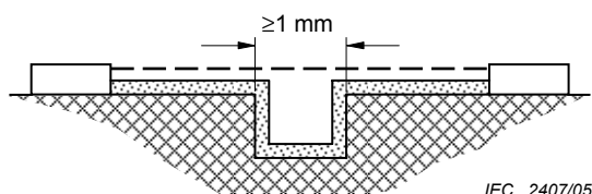
Figure 23 – LIGNE DE FUIITE et DISTANCE DANS L'AIR – Exemple 2
