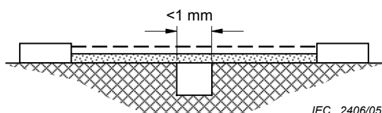
Figure 22 – LIGNE DE FUIITE et DISTANCE DANS L'AIR – Exemple 1
