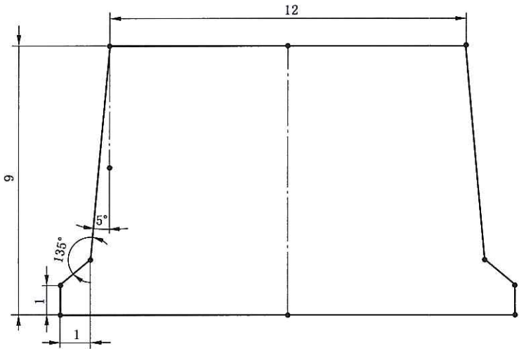
图 A.1 标准预备体模型尺寸
