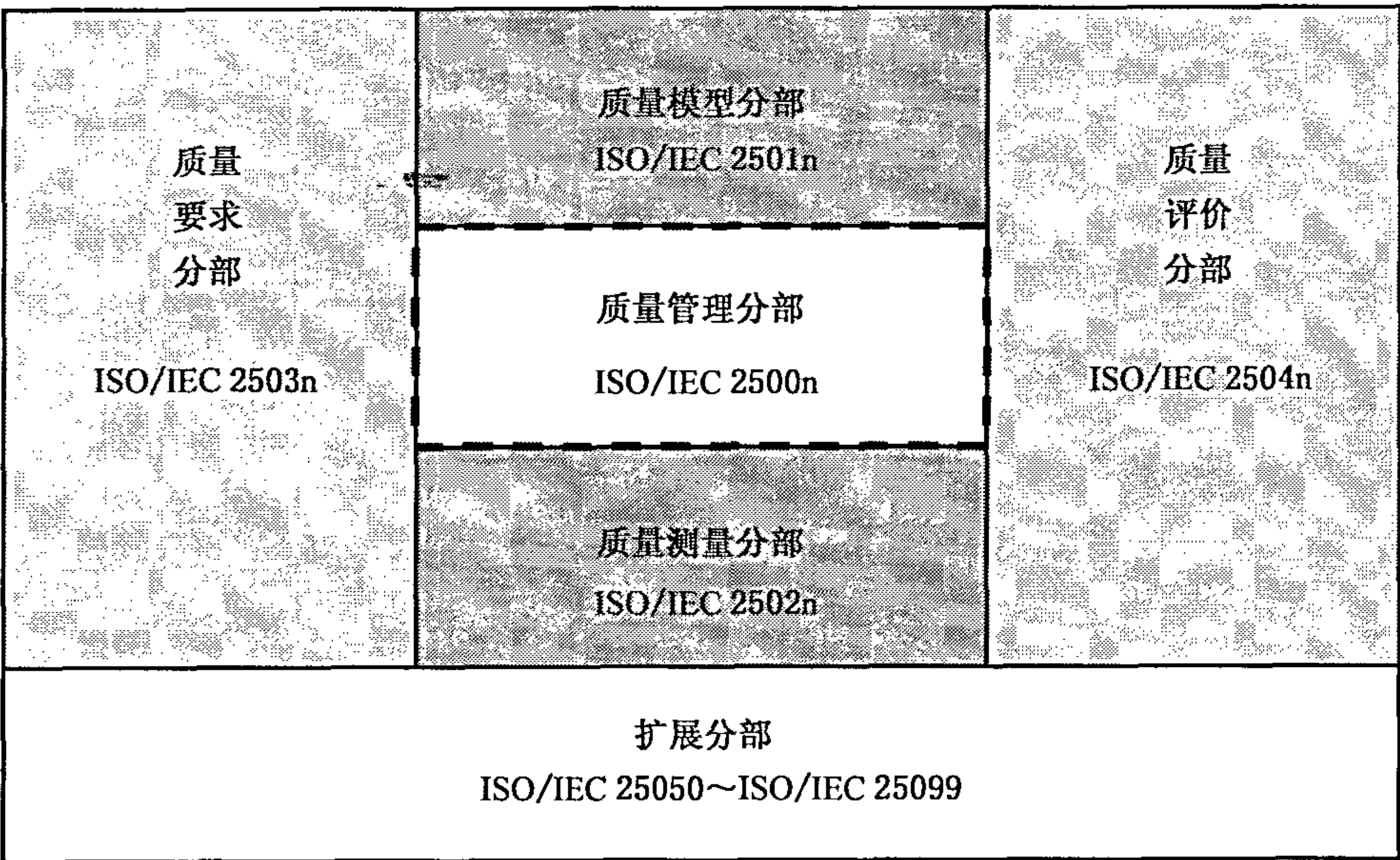
图 1 SQaRE 系列国际标准的组织
