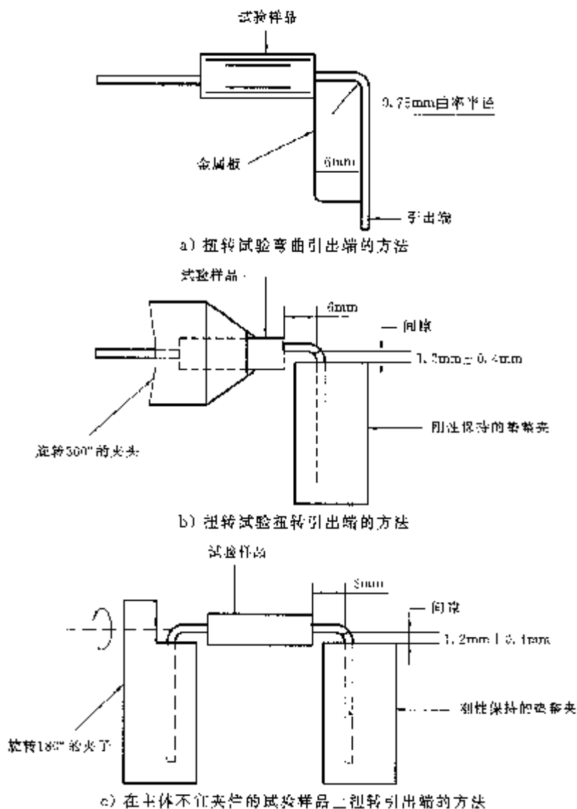
图 4 试验 Uc:线状引出端的扭转试验
