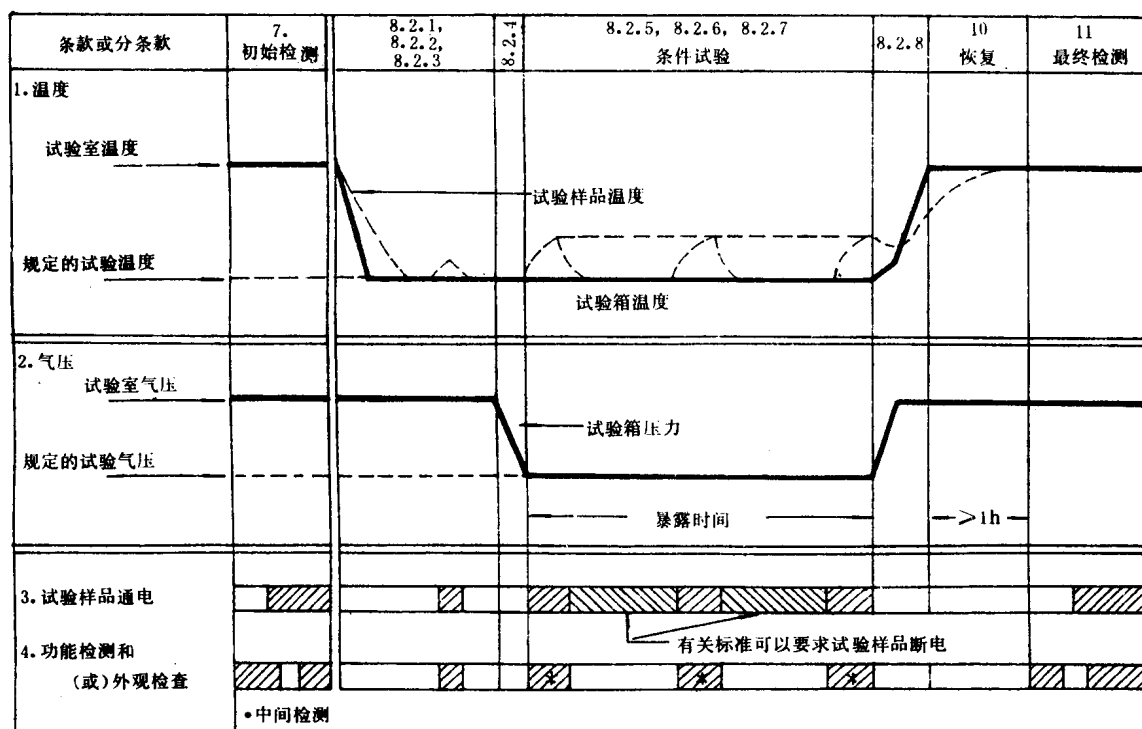
图 2 散热试验样品的试验剖面图
