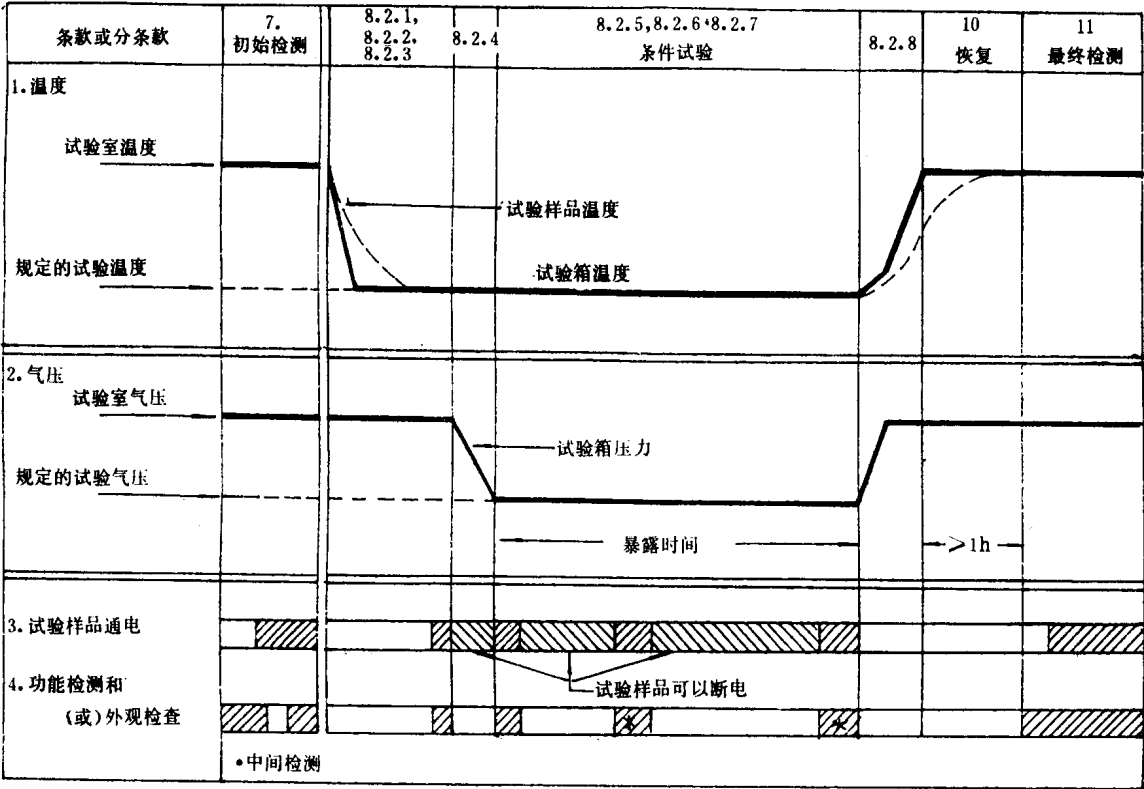
图 1 非散热试验样品的试验剖面图
