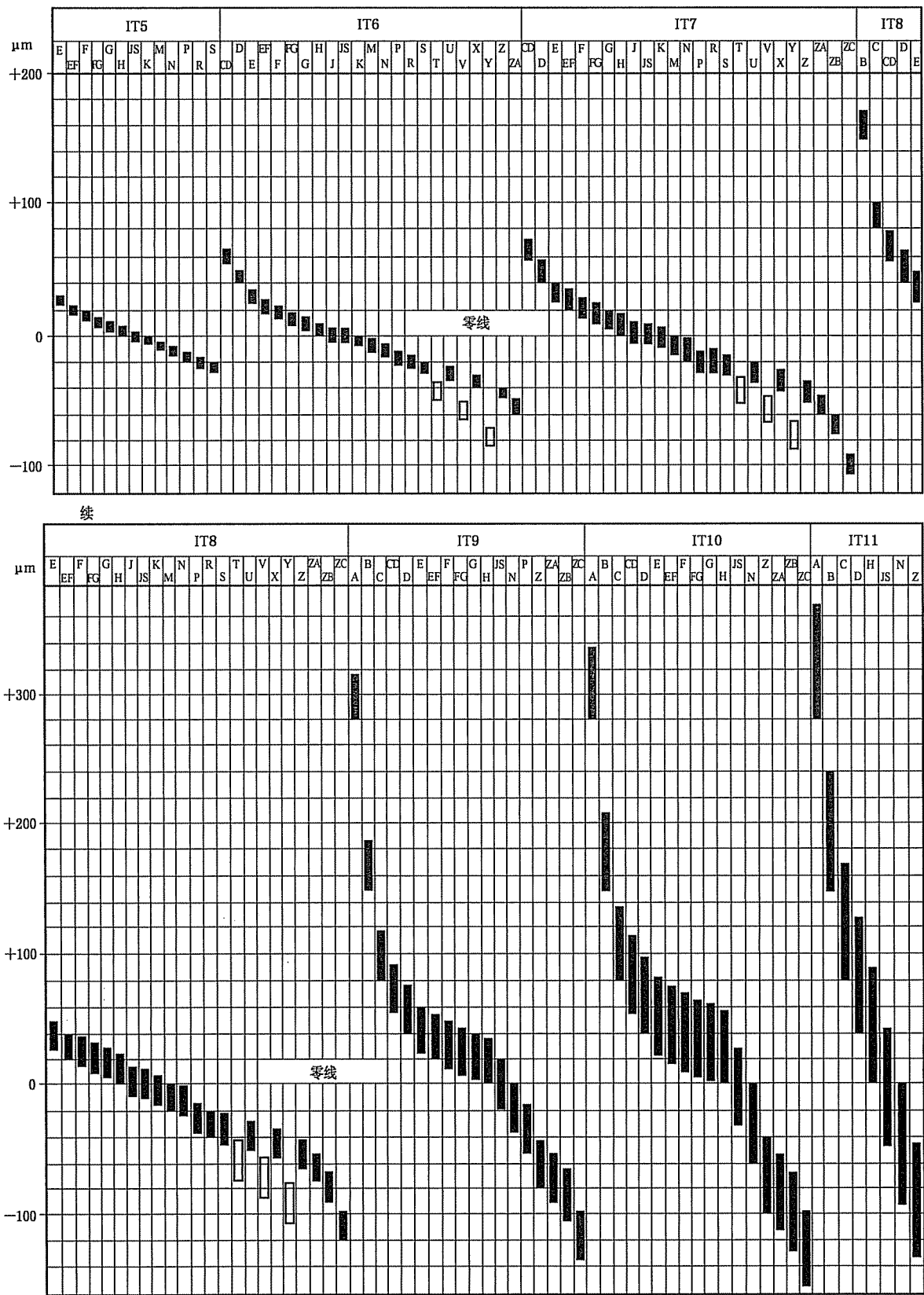
图 A.2 以公差等级图示的孔公差带
