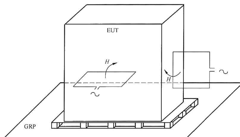
图 6 用邻近法探测磁场敏感性
