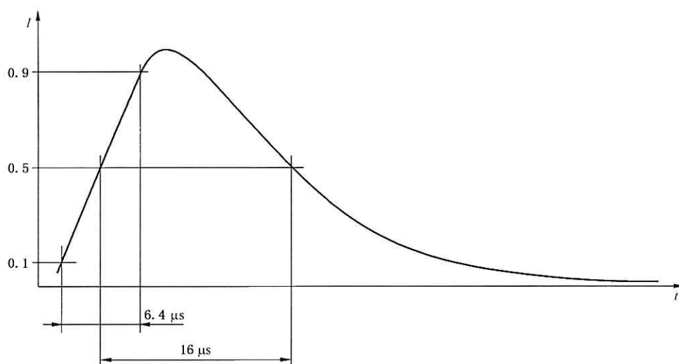
图 2 脉冲磁场试验发生器的输出电流波形(6.4/16 \mu\text{s} )
