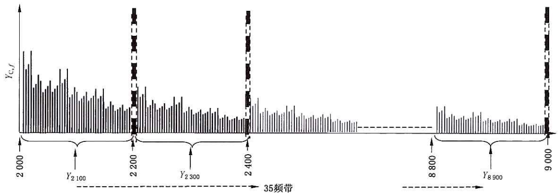
图 B.1 50 Hz 电力系统中 40 次谐波频率以上至 9 kHz 的频带范围内测量示意图
