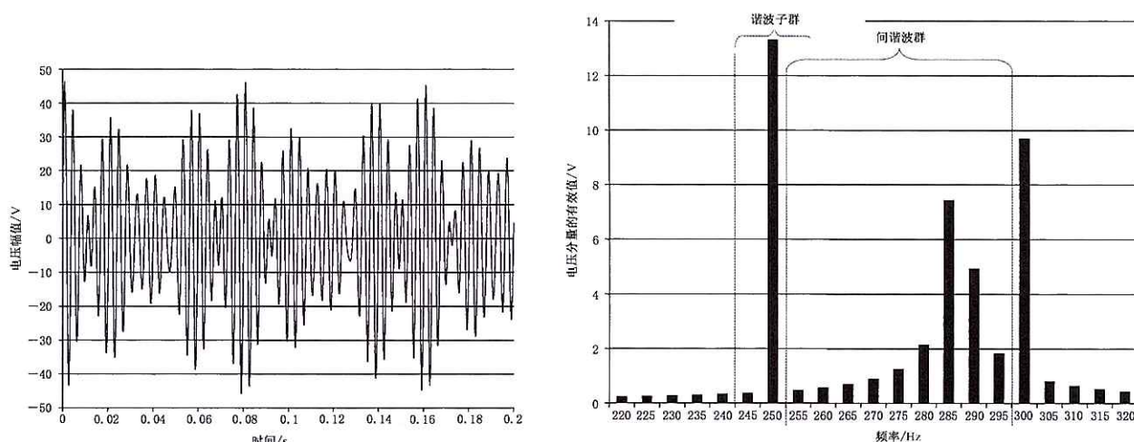
图 C.5 287 Hz 的间谐波以及 5 次和 6 次谐波
