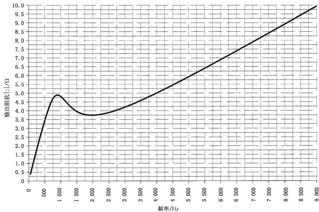
图 B.4 从 EUT 侧看人工电源网络阻抗
