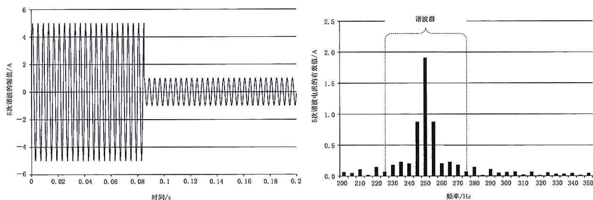
图 C.1 5 次谐波电流大波动
