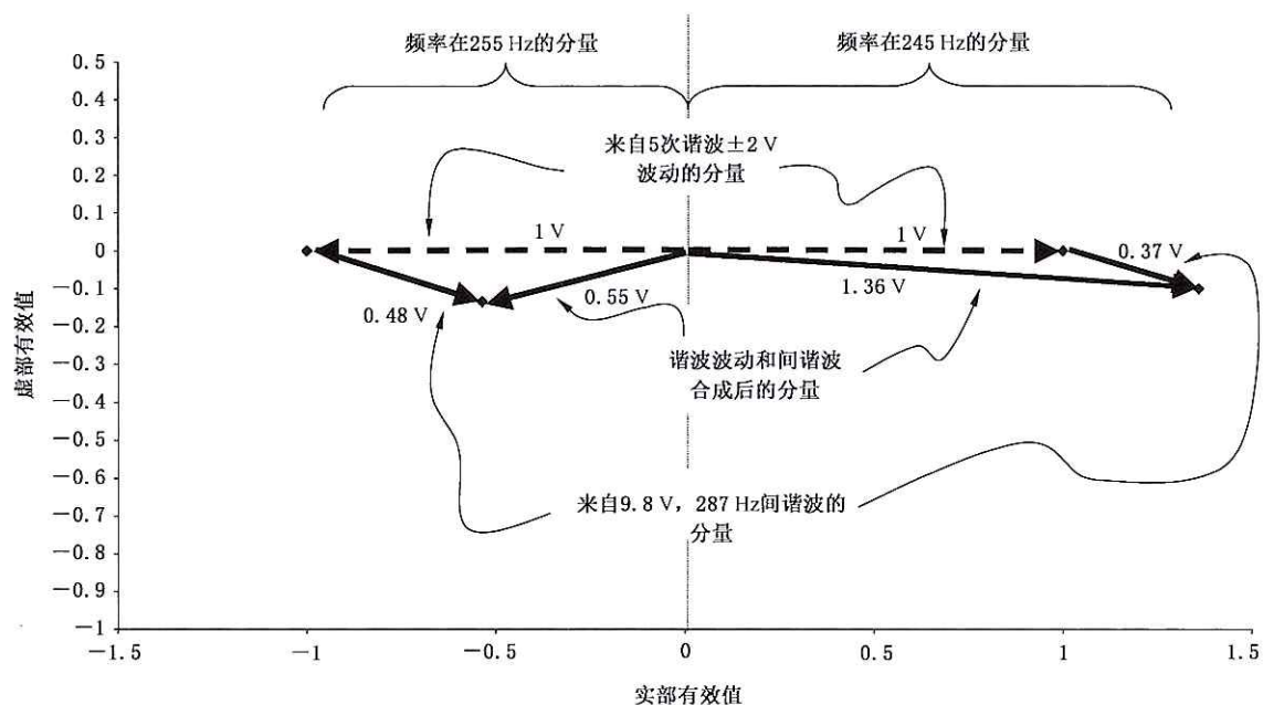
图 C.7 频率分别为 245 Hz 和 255 Hz 处的矢量
