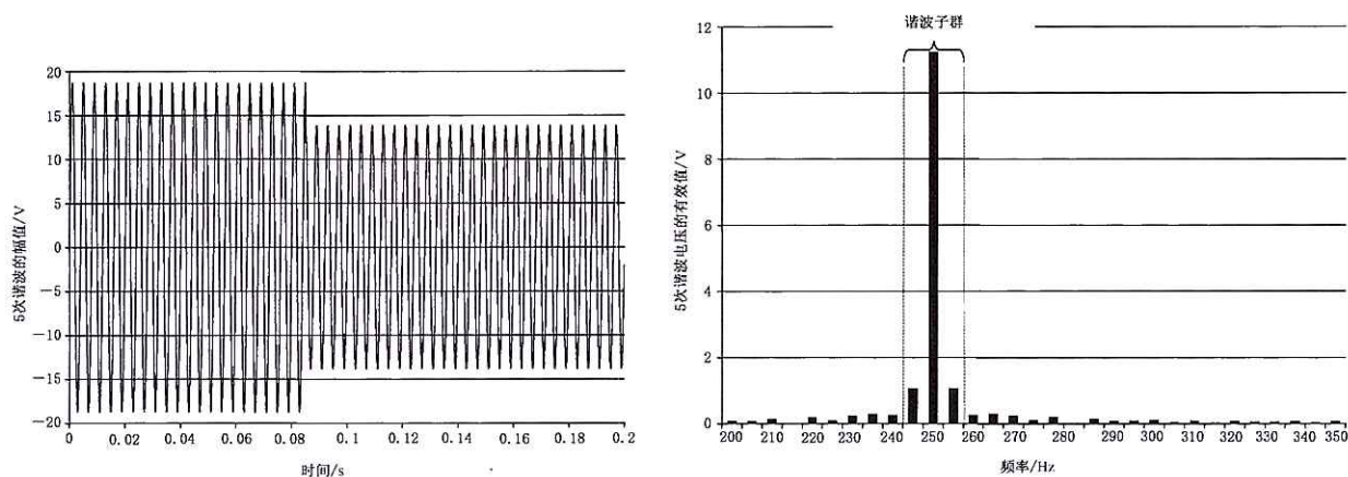
图 C.2 5 次谐波电压大波动
