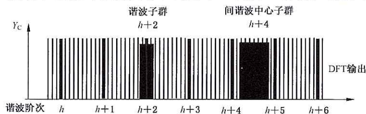
图 6 谐波子群和间谐波中心子群示例(图示为 50 Hz 电源)
