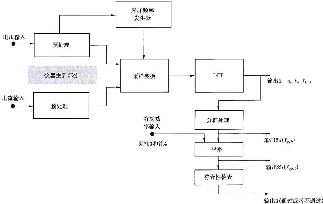
图 1 测量仪器的通用架构
