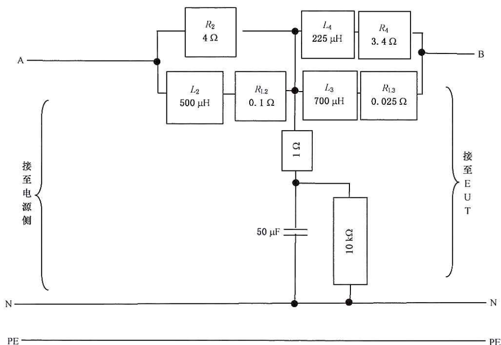
图 B.3 适用于 16 A 电流及以下测量的人工电源网络
