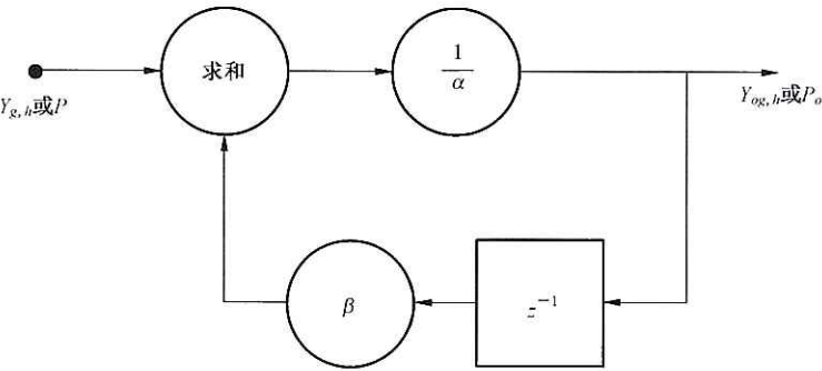
图 5 数字低通滤波器的实现原理[ z^{-1} 表示时间窗延迟, \alpha 、 \beta 为滤波器系数(数值见表 2)]
