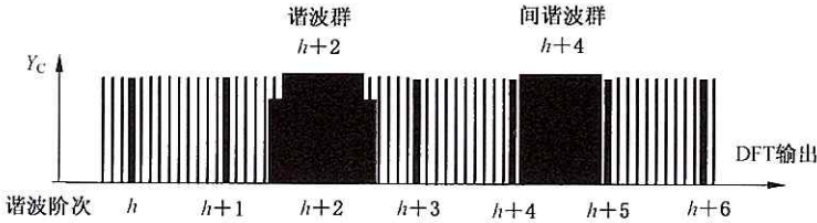
图 4 谐波群和间谐波群示意图(图示为 50 Hz 电源)
