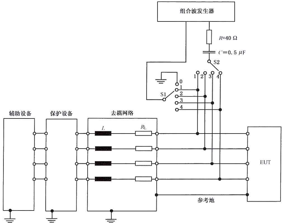
图 10 交流线(三相)上电容耦合的试验配置示例;线 L3-地耦合(见 7.2)
