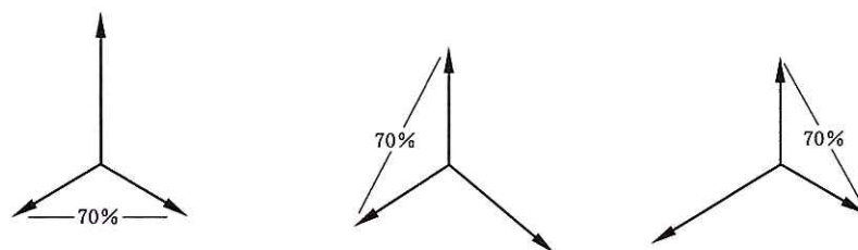
d) 不可接受的方法——相线对相线无相移试验
