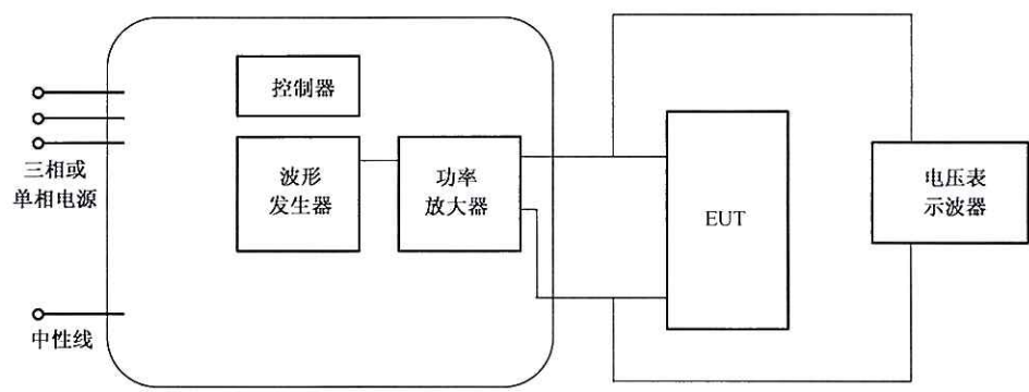
图 3 带有功率放大器的试验仪器的原理图
