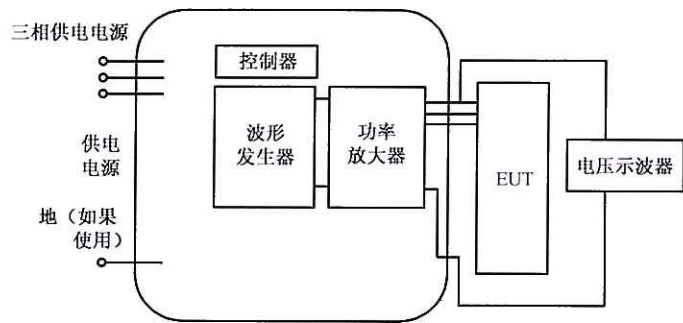
图 3 不平衡试验装置的示意图
