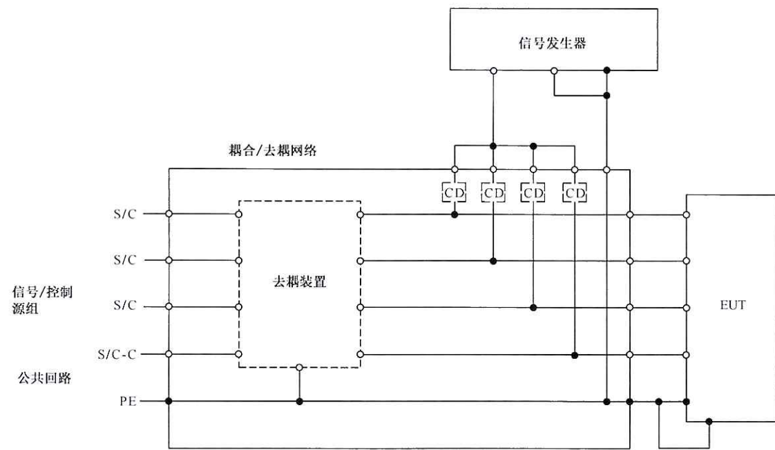
b) 使用专用接地连线的试验布置
