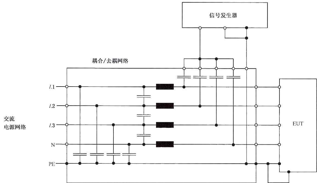
a) 使用接地参考平面的试验布置
