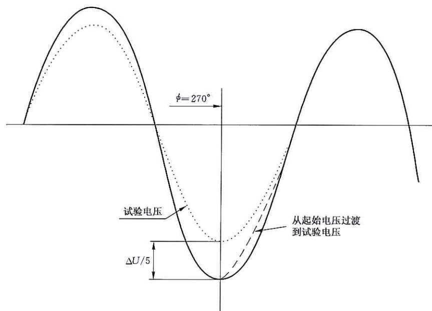
b) t_f 和 t_r 等于 0.25 周期阶跃电压的例子
