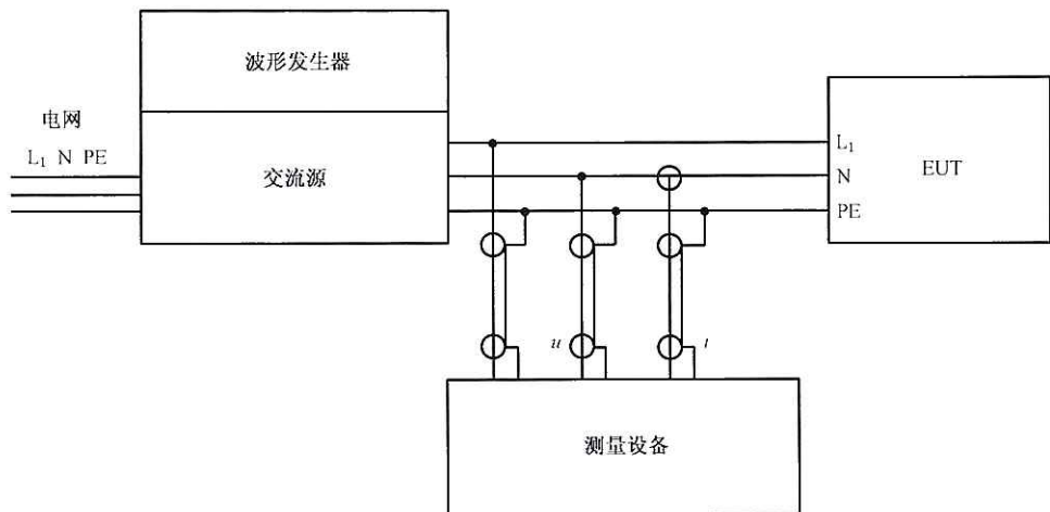
图 2 单相 EUT 试验布置举例
