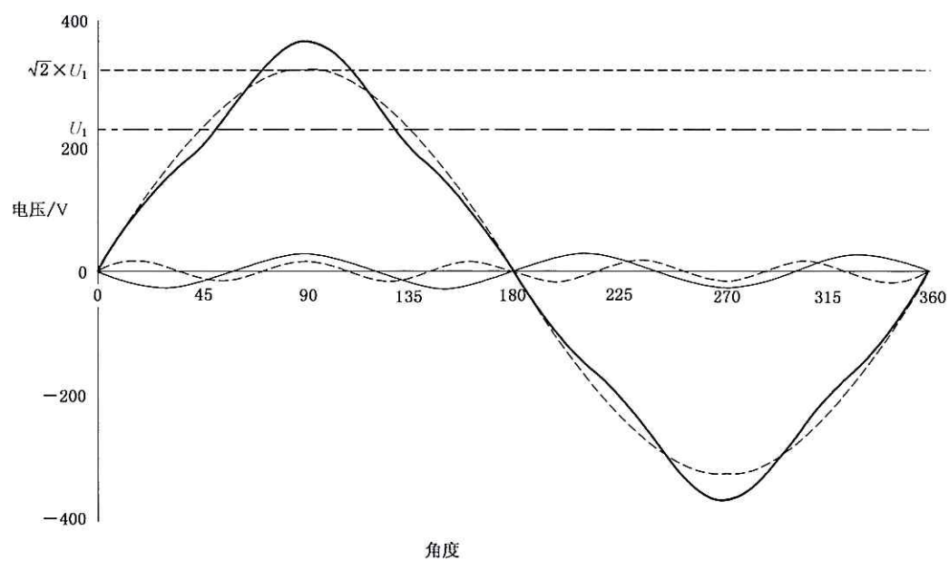
图 7 尖顶波波形
