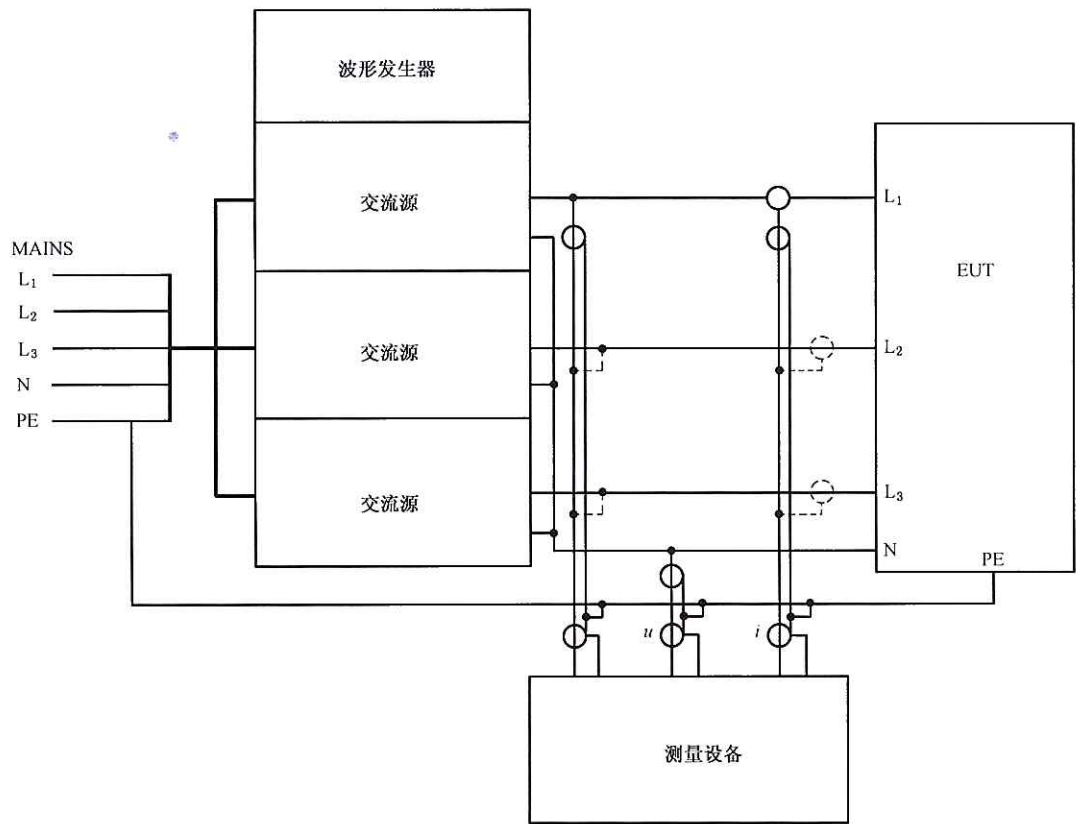
图 3 三相 EUT 试验布置举例
