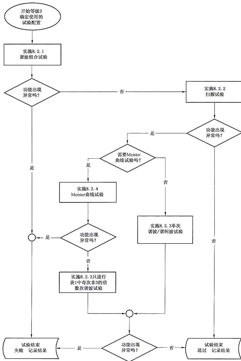
图 1b) 等级 3 的试验流程图
