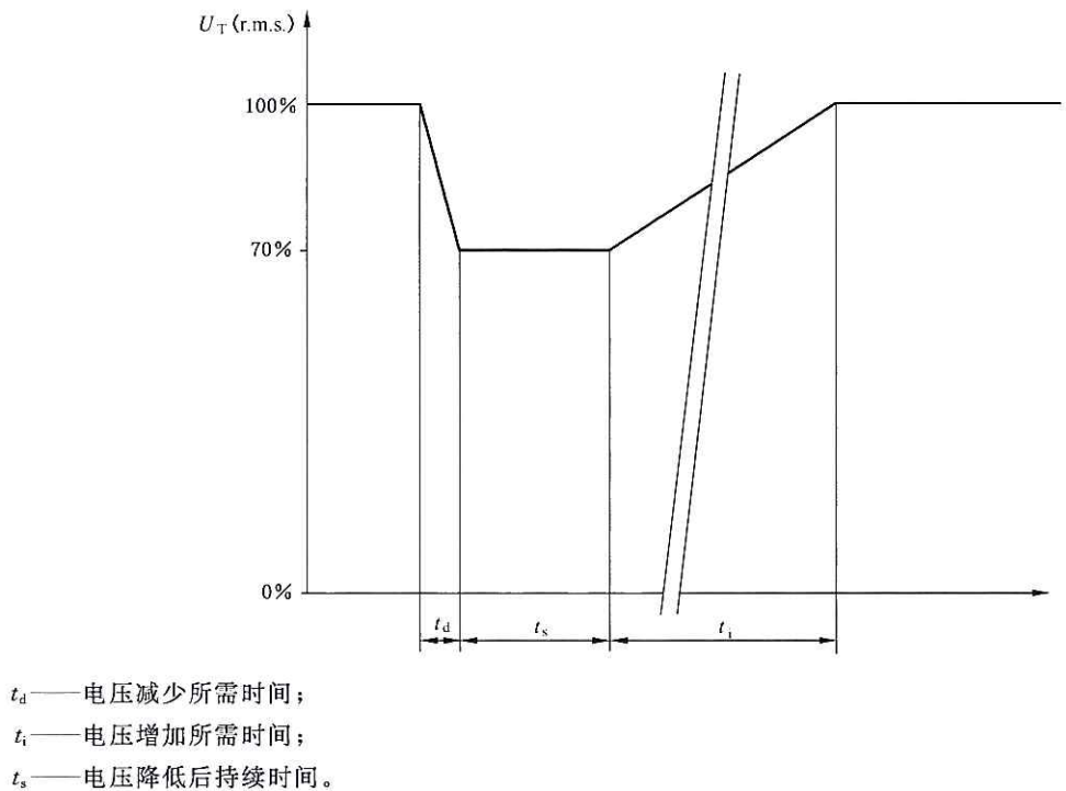
图 3 电压变化
