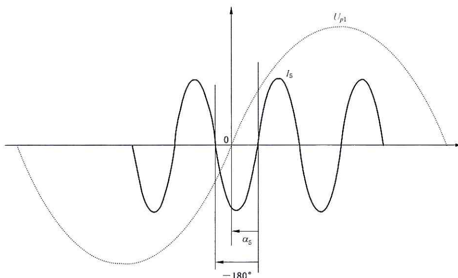
图2 第5次谐波电流相角的定义($I_5$ 滞后 $U_{p1}$, $\alpha_5 &lt; 0$)
