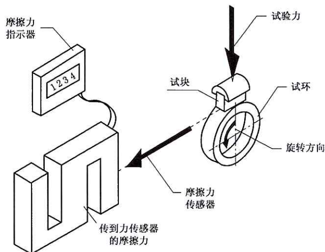
图3 试验基本装置示意图
