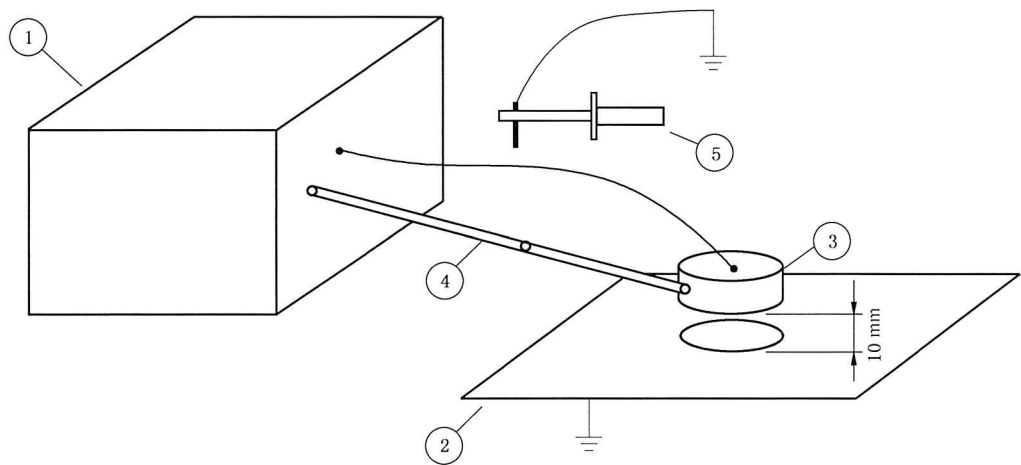
图 201.102 测试探头
