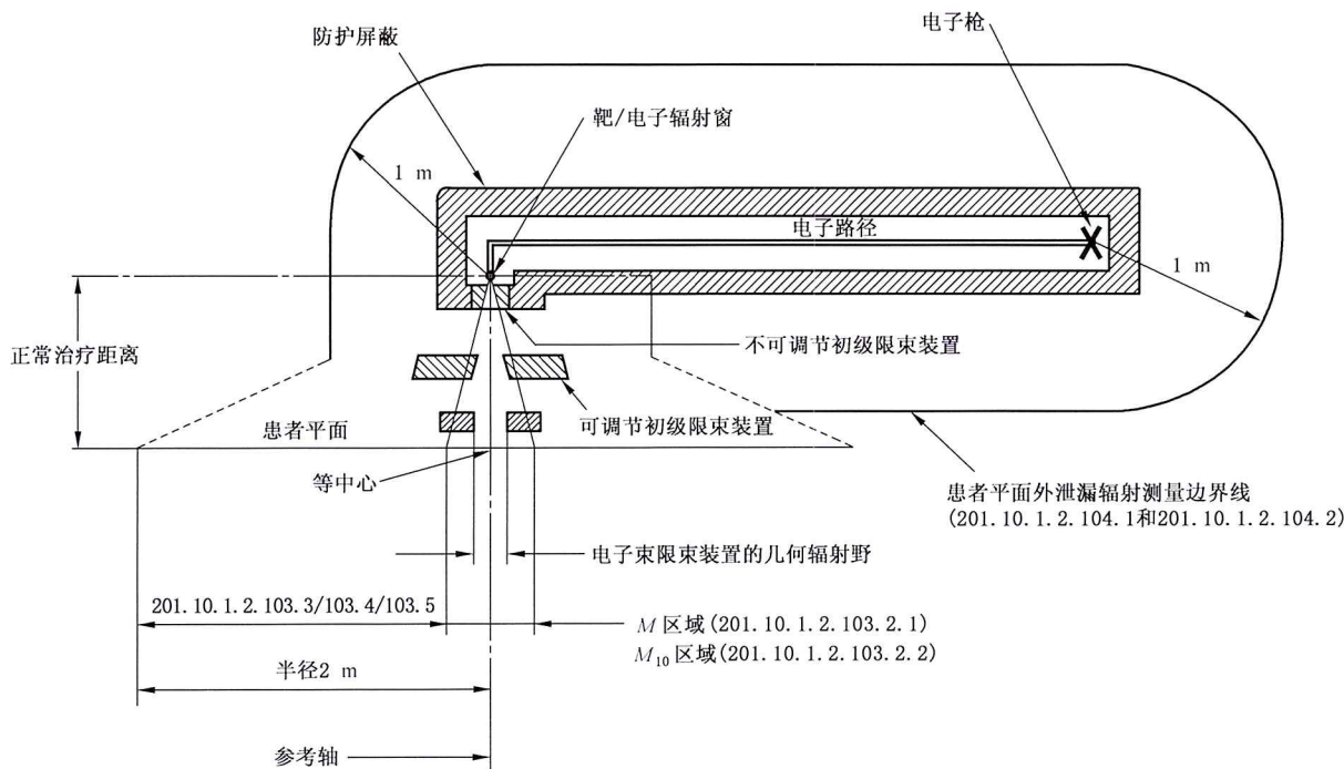
图 201.103 正视图——用于泄漏辐射要求(201.10.1.2.103 和 201.10.1.2.104)
