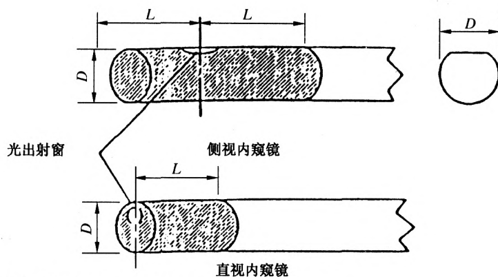
图 101 光出射部分图
