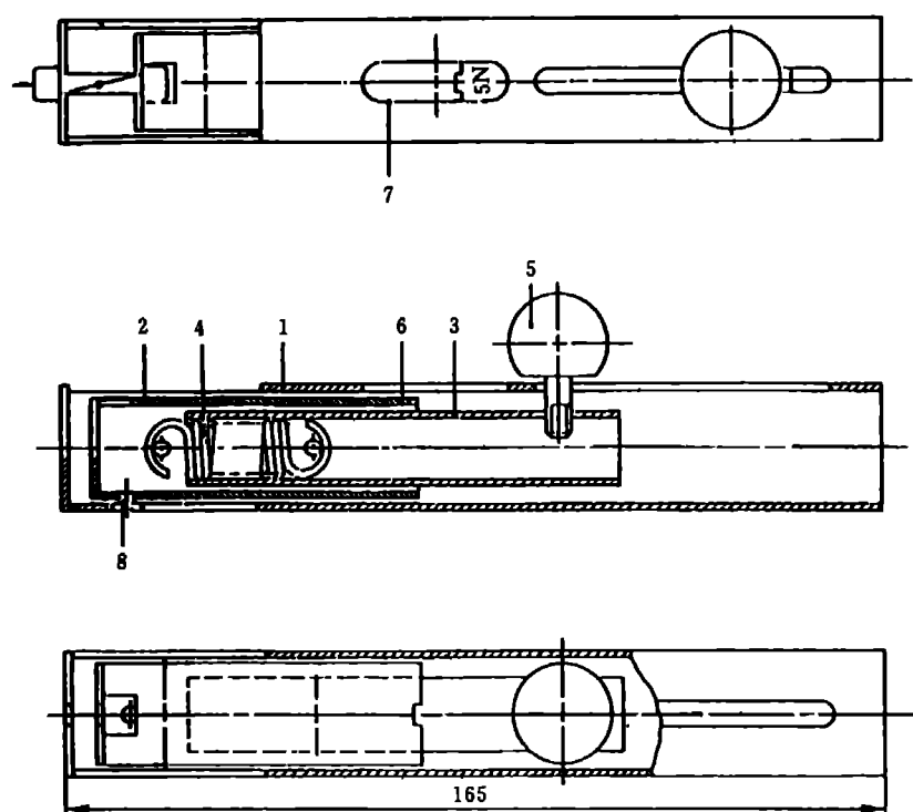
图 7 轴向拉力试验装置
