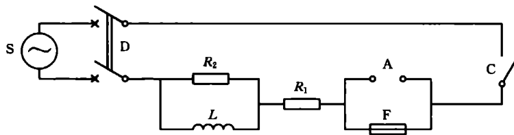
图5 高分断能力熔断体分断能力试验典型电路(见9.3)
