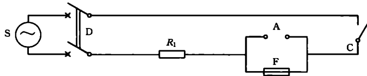
图6 低分断能力熔断体分断能力试验典型电路(见9.3)
