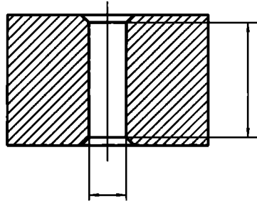
图4 准直度标准规(见8.4)
