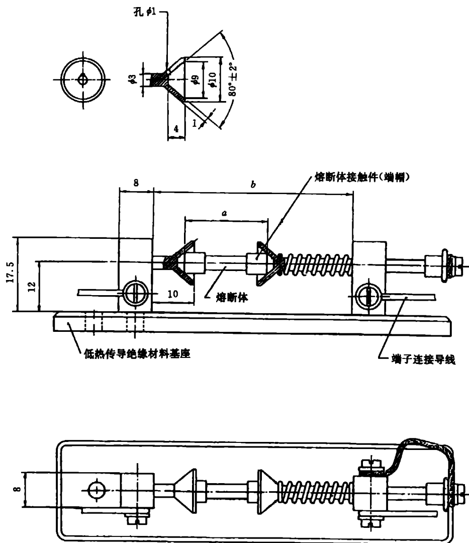
图1 5mm×20mm 和 6.3×3.2mm 熔断体试验用熔断器座 额定电流不大于 10A(见 7.3.1)
