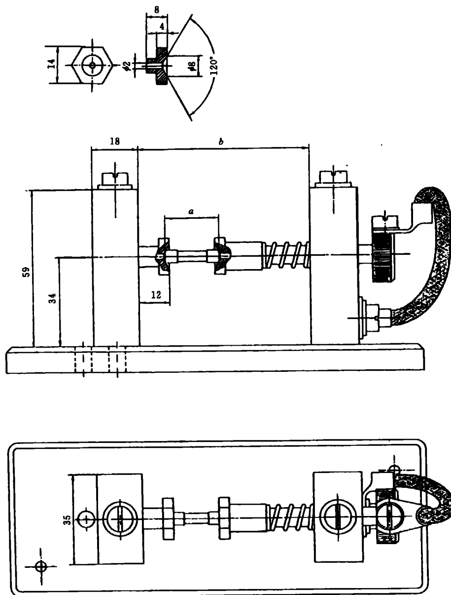
图3 分断能力试验用熔断器座(见 7.3.1)
