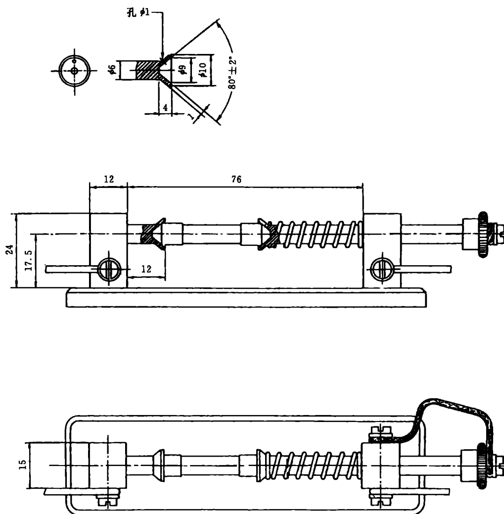
图 2 6.3mm×3.2mm 熔断体试验用熔断器座 额定电流大于 10A(见 7.3.1)
