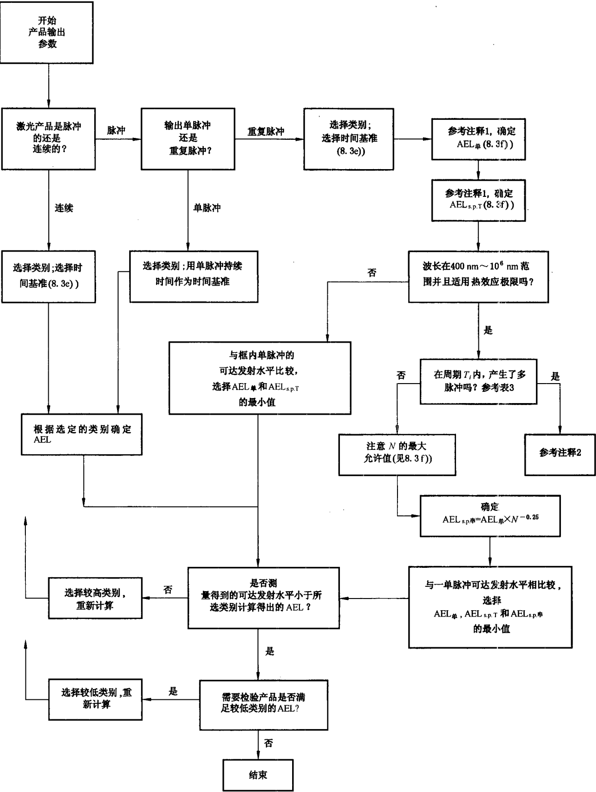
图 B.1 根据提供的输出参数,对激光产品进行分类的流程图
