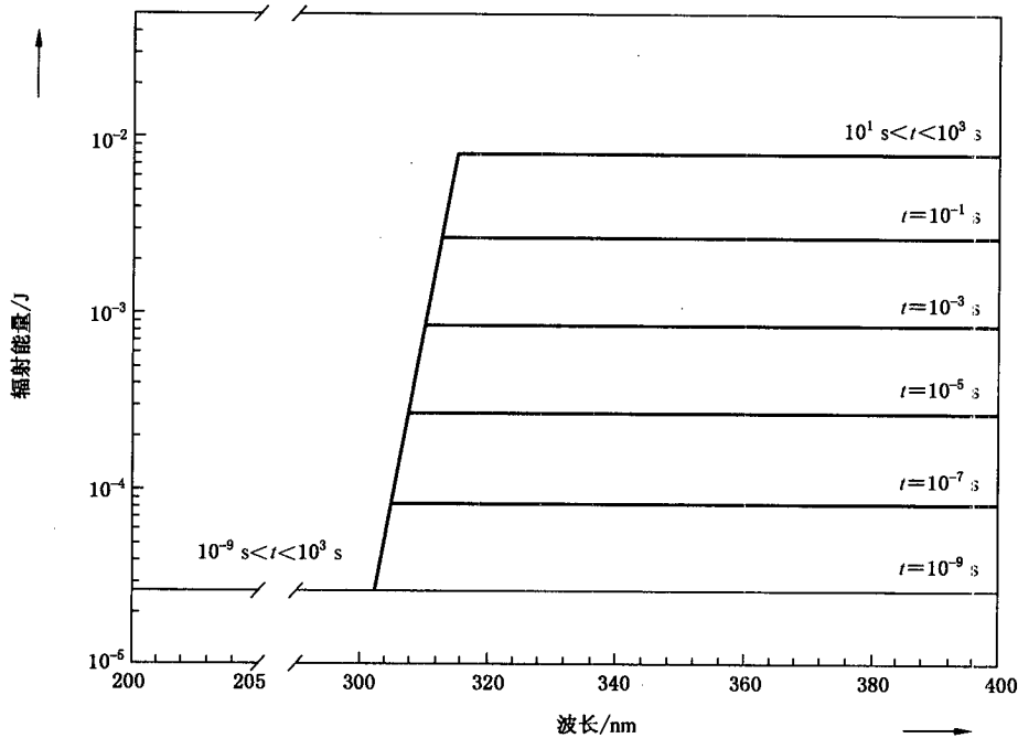
图 B.3 对选定发射持续时间 10^{-9} \text{ s} \sim 10^3 \text{ s} 的 1 类紫外激光产品的 AEL 值
