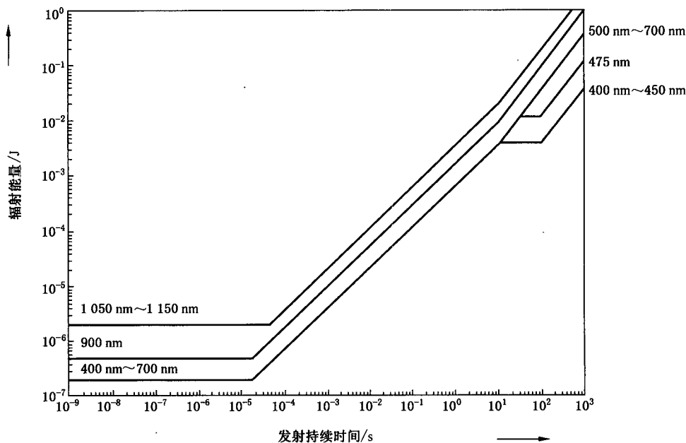
图 B.5 1 类可见和选定红外激光产品的 AEL 值( C_6 = 1 )
