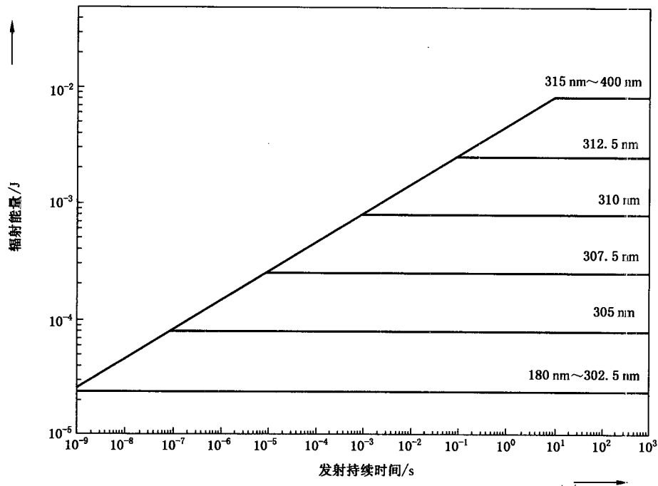
图 B.4 在选定波长上,发射持续时间 10^{-9} \text{ s} \sim 10^3 \text{ s} 的 1 类紫外激光产品的 AEL 值
