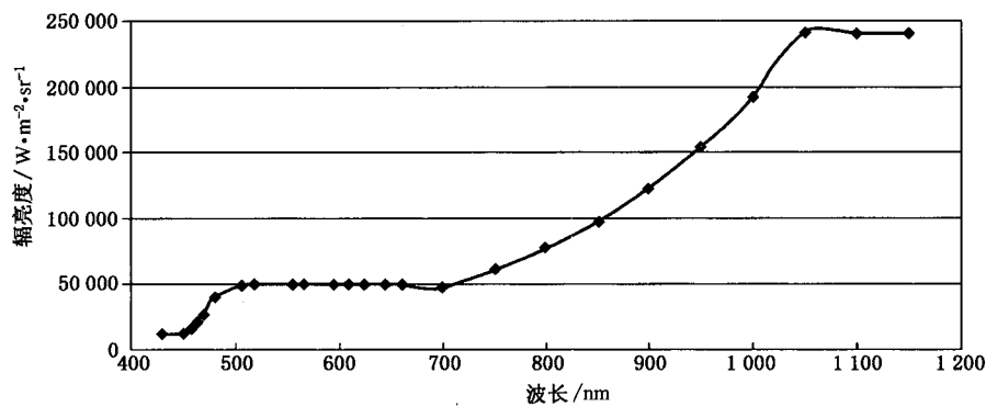
图 E.1 辐亮度是波长的函数
