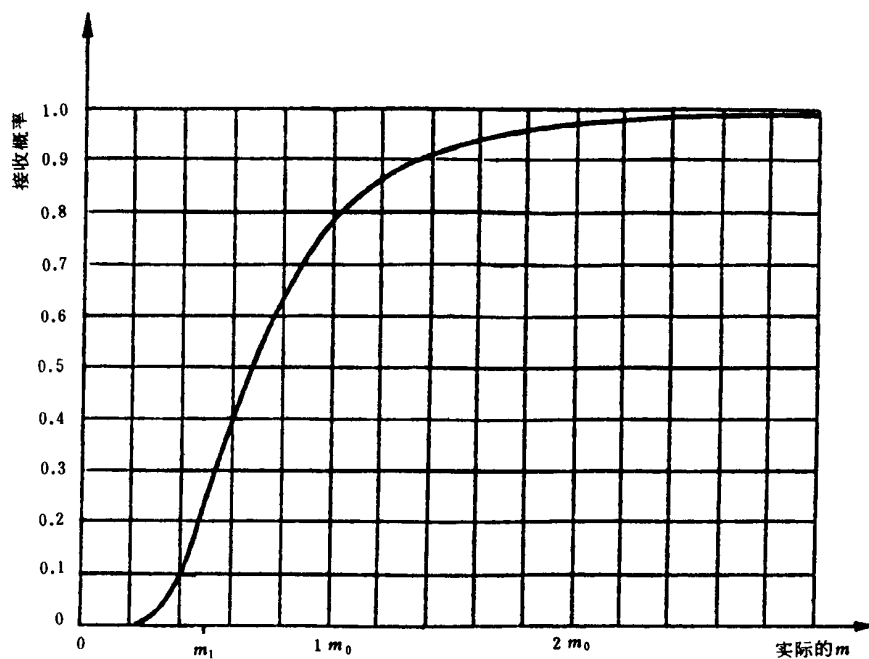
图 18 试验方案4:6工作特性曲线
