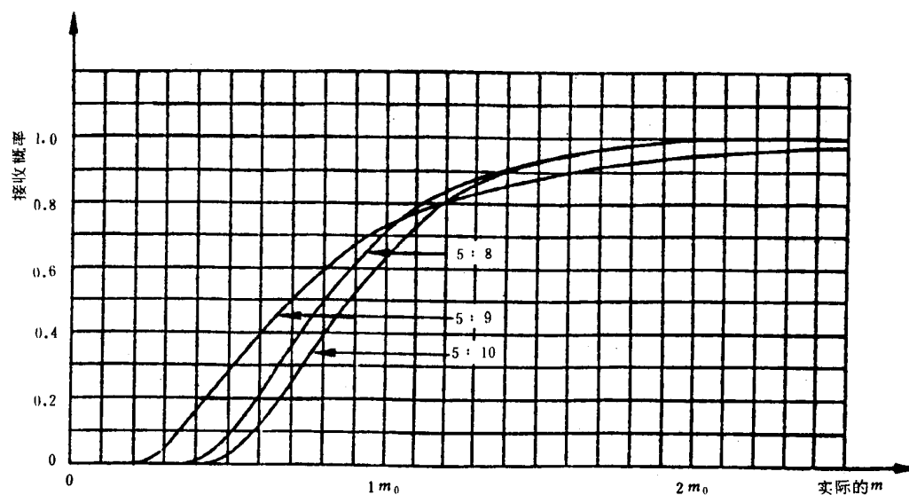
图 41 试验方案5:8, 5:9和5:10工作特性曲线
