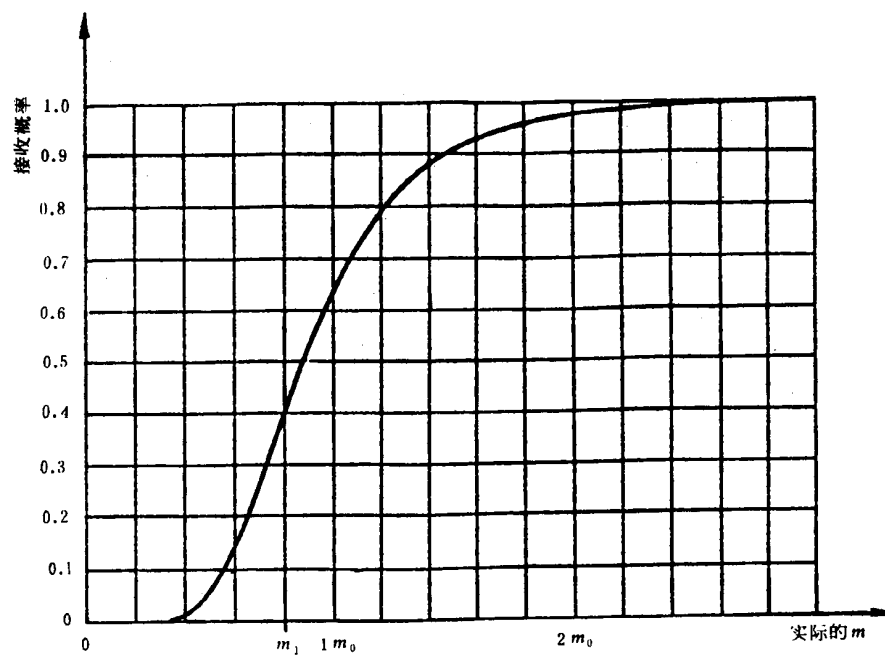
图 30 试验方案4:10工作特性曲线
