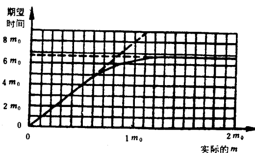
图 44 试验方案5:10判定的期望相关试验时间
