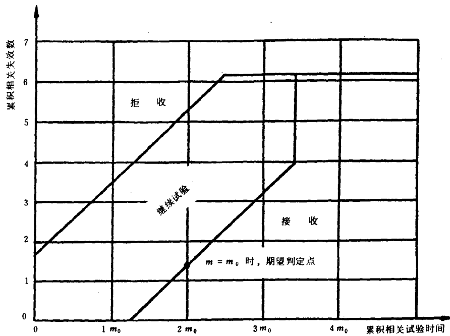
图 8 试验方案4:3 ( \alpha=0.10 , \beta=0.10 , D_m=3.0 )
