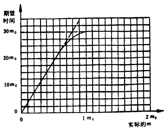
图 33 试验方案5:1判定的期望相关试验时间
