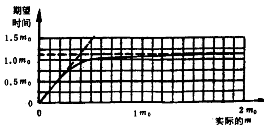
图 36 试验方案5:4判定的期望相关试验时间
