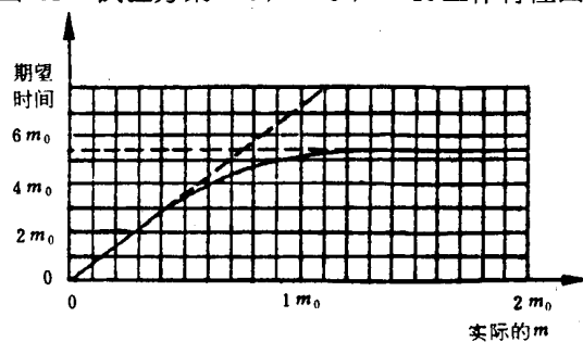
图 42 试验方案5:8判定的期望相关试验时间
