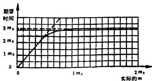
图 35 试验方案5:3判定的期望相关试验时间
