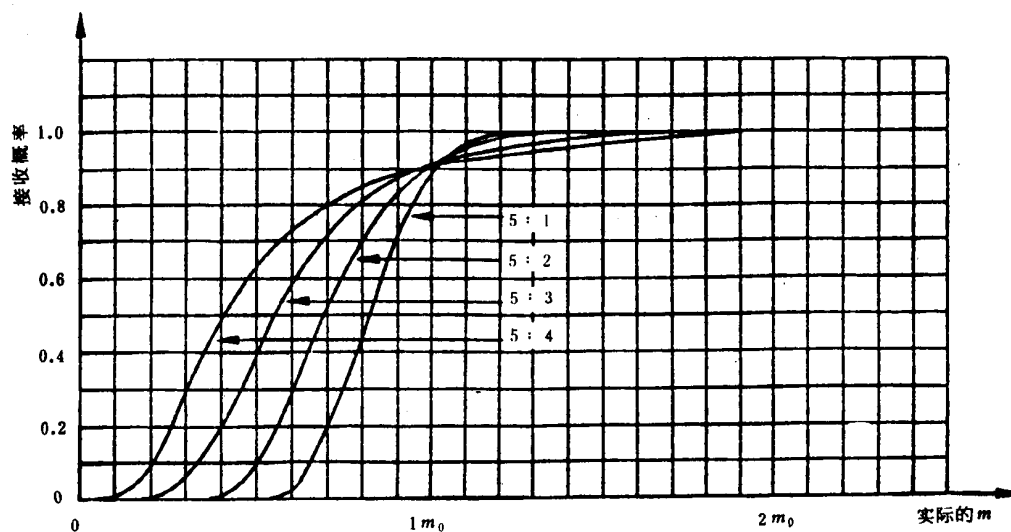
图 32 试验方案5:1, 5:2, 5:3和5:4工作特性曲线
