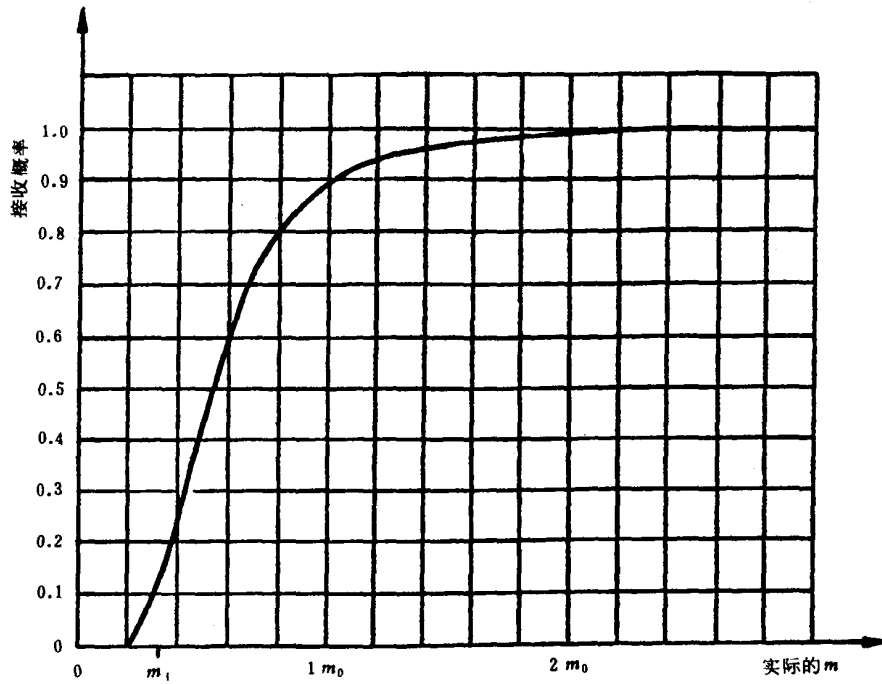
图 9 试验方案4:3工作特性曲线
