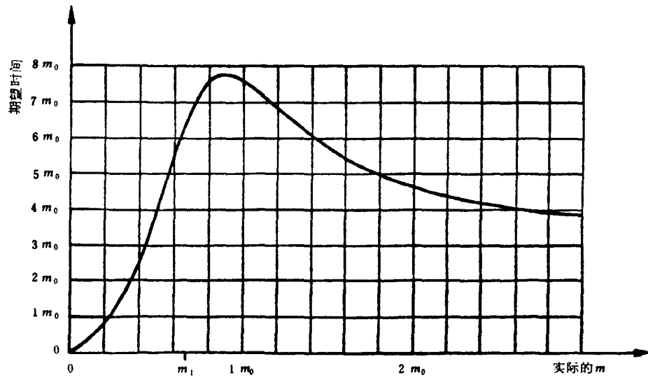
图 16 试验方案4:5判定的期望相关试验时间
