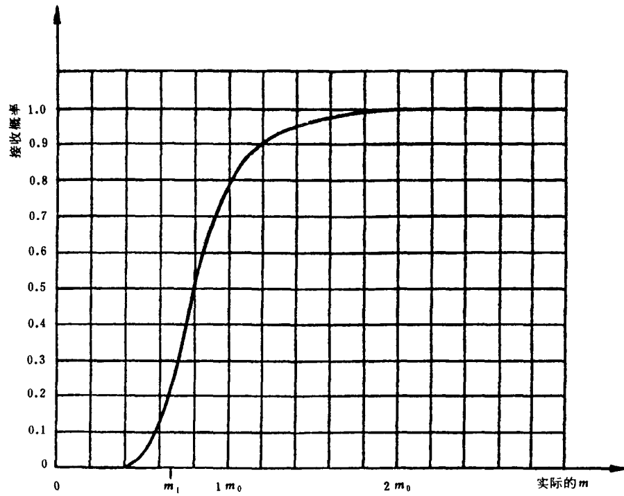
图 15 试验方案4:5工作特性曲线
