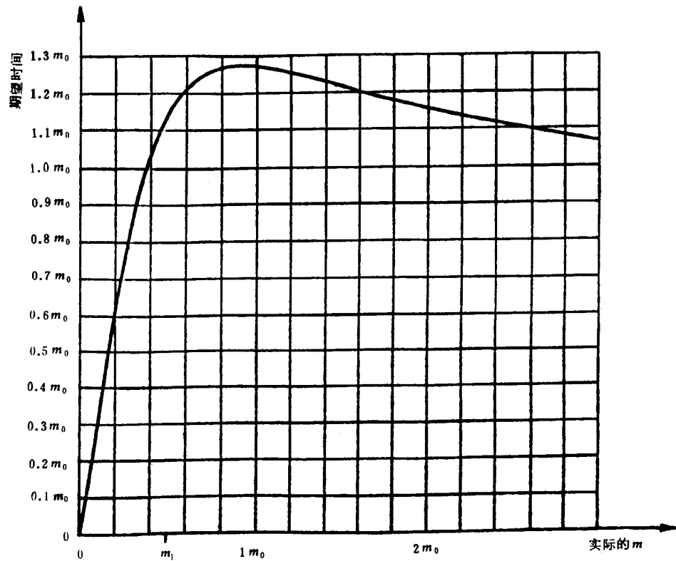
图 28 试验方案4:9判定的期望相关试验时间
