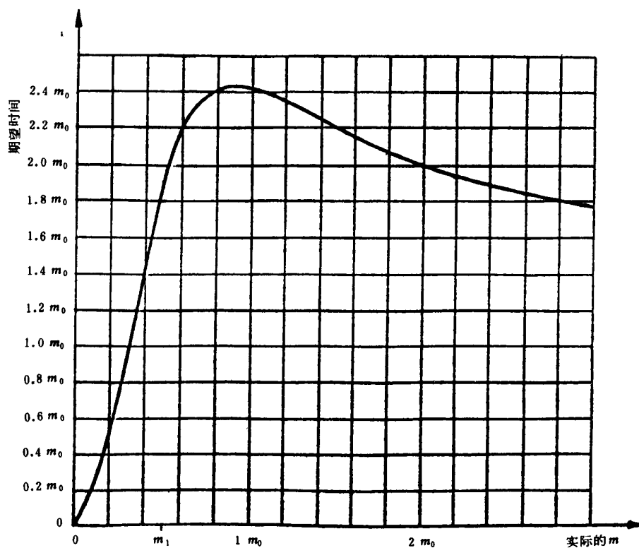
图 19 试验方案4:6判定的期望相关试验时间
