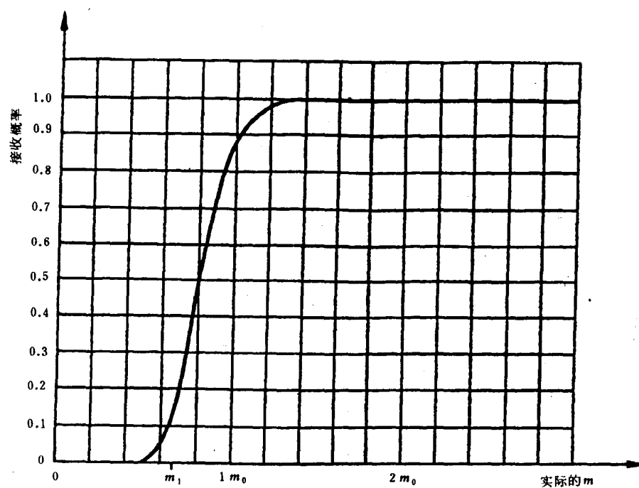
图 3 试验方案4:1工作特性曲线
