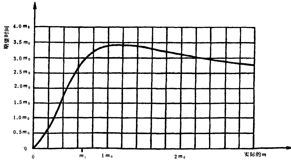
图 24 试验方案4:8工作特性曲线
