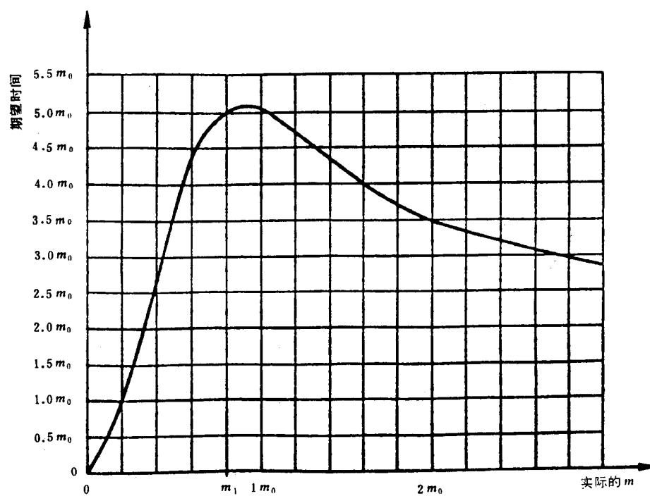
图 31 试验方案4:10判定的期望相关试验时间
