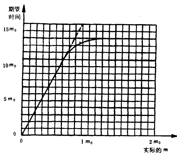
图 38 试验方案5:5判定的期望相关试验时间
