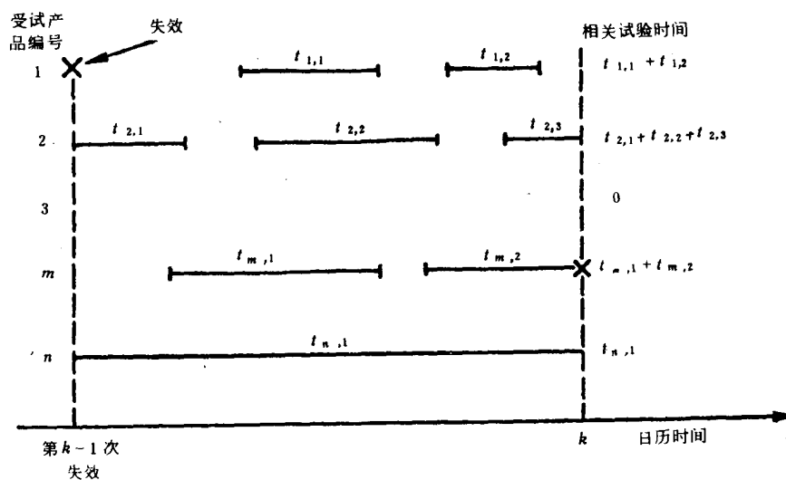
图 1 相关试验时间的周期编号
