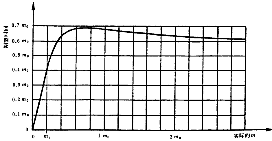
图 13 试验方案4:4判定的期望相关试验时间
