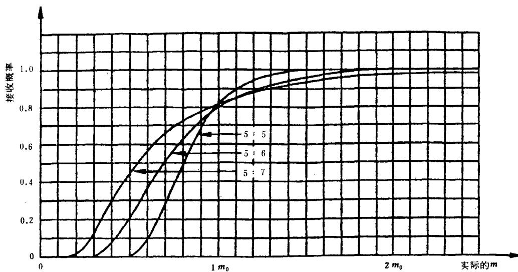
图 37 试验方案5:5, 5:6, 5:7工作特性曲线
