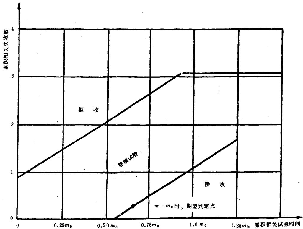
图 11 试验方案4:4 ( \alpha=0.10 , \beta=0.10 , D_m=5.0 )
