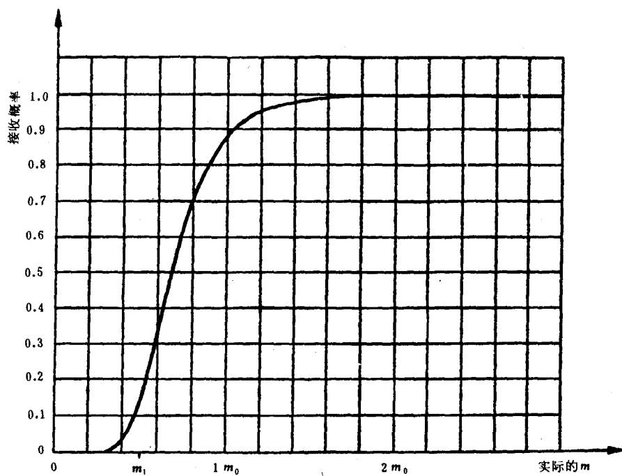
图 6 试验方案4:2工作特性曲线
