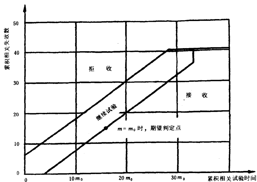
图 2 试验方案4:1 ( \alpha=0.10 , \beta=0.10 , D_m=1.5 )
