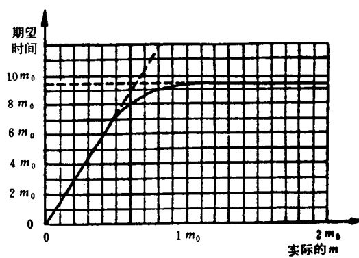
图 34 试验方案5:2判定的期望相关试验时间
