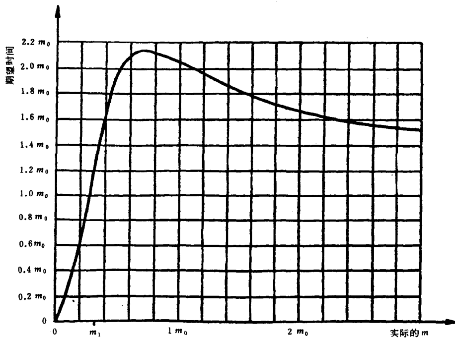
图 10 试验方案4:3判定的期望相关试验时间
