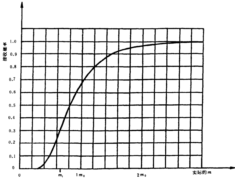
图 24 试验方案4:8工作特性曲线
