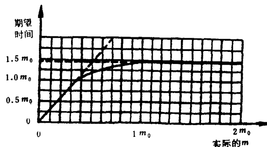
图 40 试验方案5:7判定的期望相关试验时间
