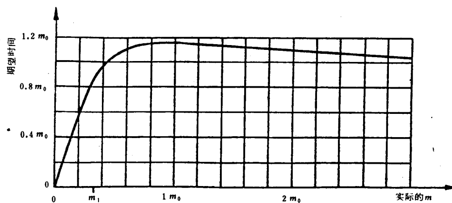
图 22 试验方案4:7 判定的期望相关试验时间
