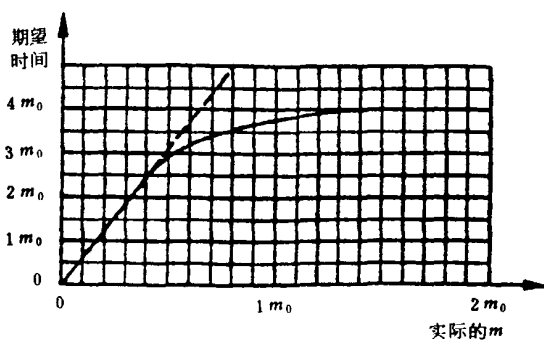
图 39 试验方案5:6判定的期望相关试验时间
