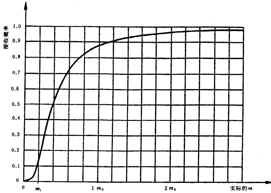
图 12 试验方案4:4工作特性曲线
