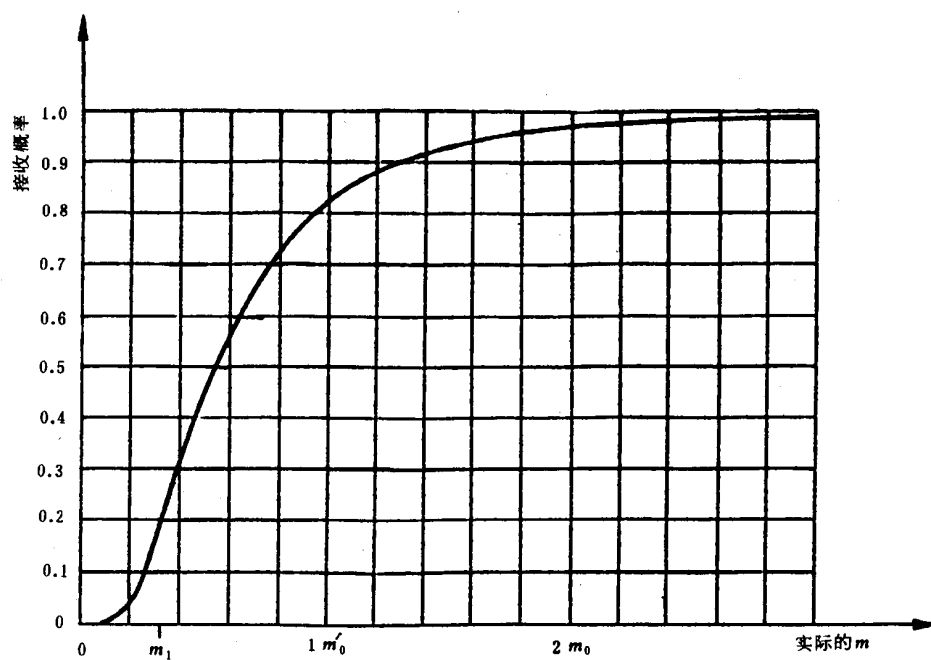
图 21 试验方案4:7 工作特性曲线
