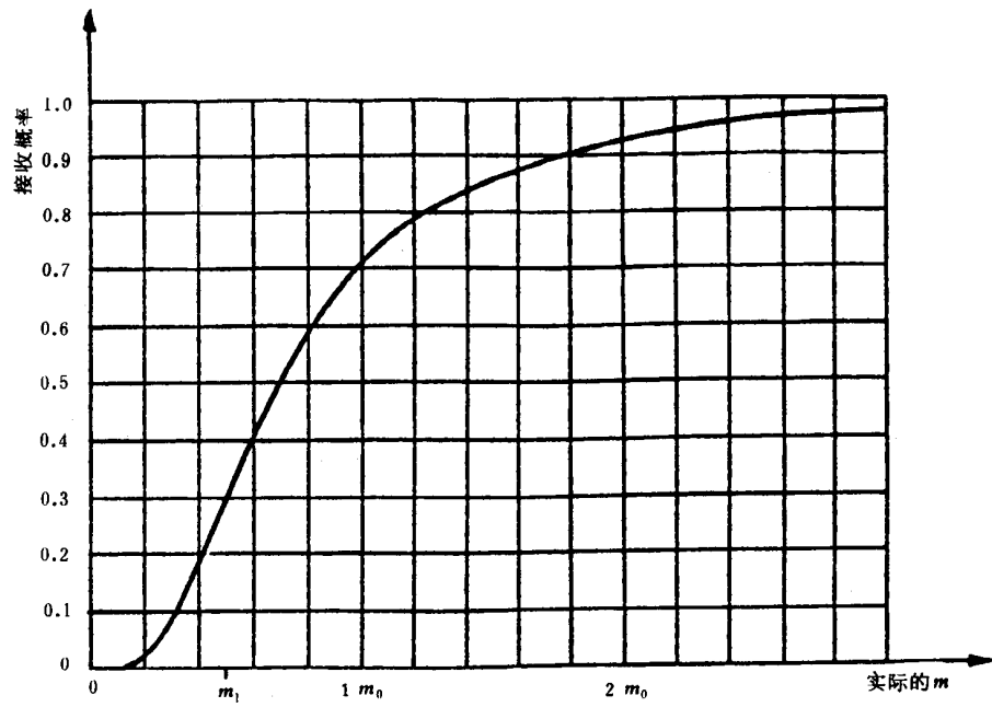
图 27 试验方案4:9工作特性曲线
