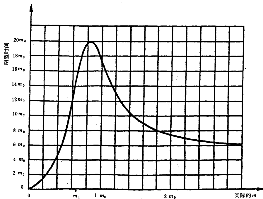
图 4 试验方案4:1判定的期望相关试验时间
