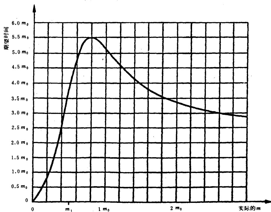
图 7 试验方案4:2判定的期望相关试验时间
