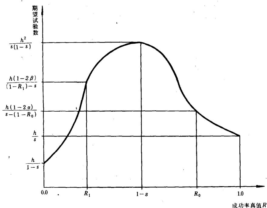
图 3 期望试验数曲线
