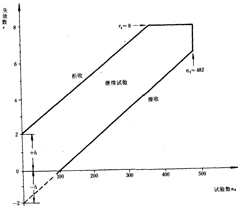
图 1 截尾序贯试验示例
