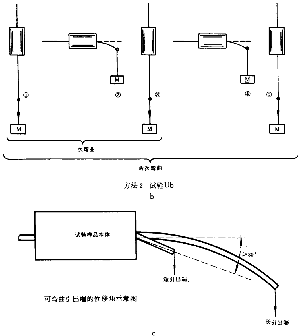
图 2 试验 Ub: 弯曲试验的试验程序示意图 (见 3.4.2.1 和 3.4.2.3 项)
