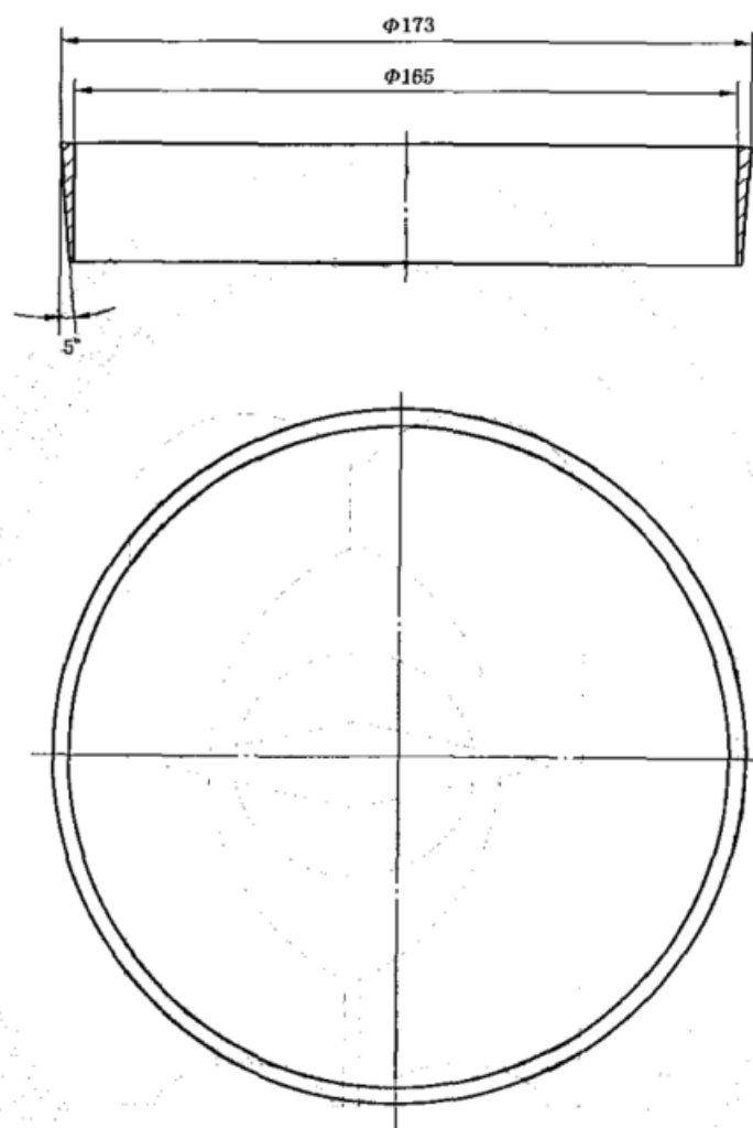
图 A.2 内环
