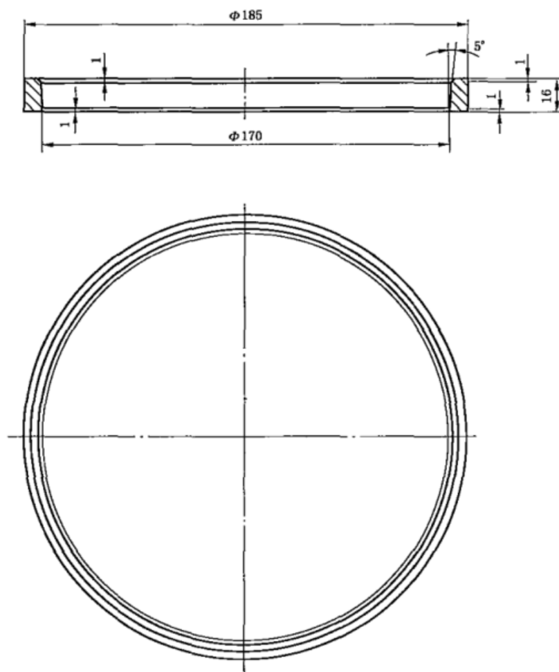
图 A.3 外环
