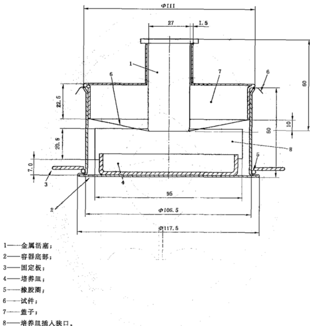
图2 试验容器
