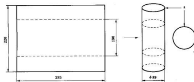
图4 试件
