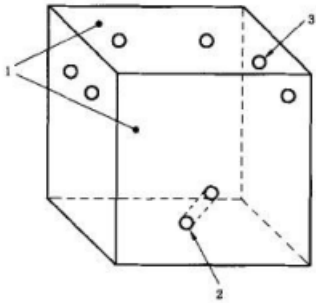
图 1 Geblo 扭曲干态微粒发生器
