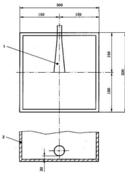
图 3 空气采样口的位置
