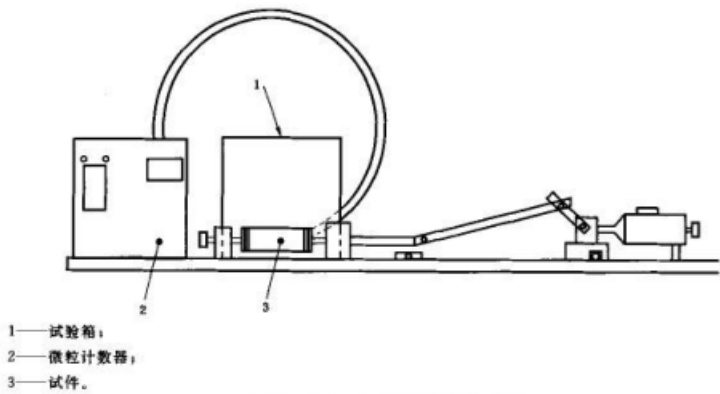
图 1 Geblo 扭曲干态微粒发生器
