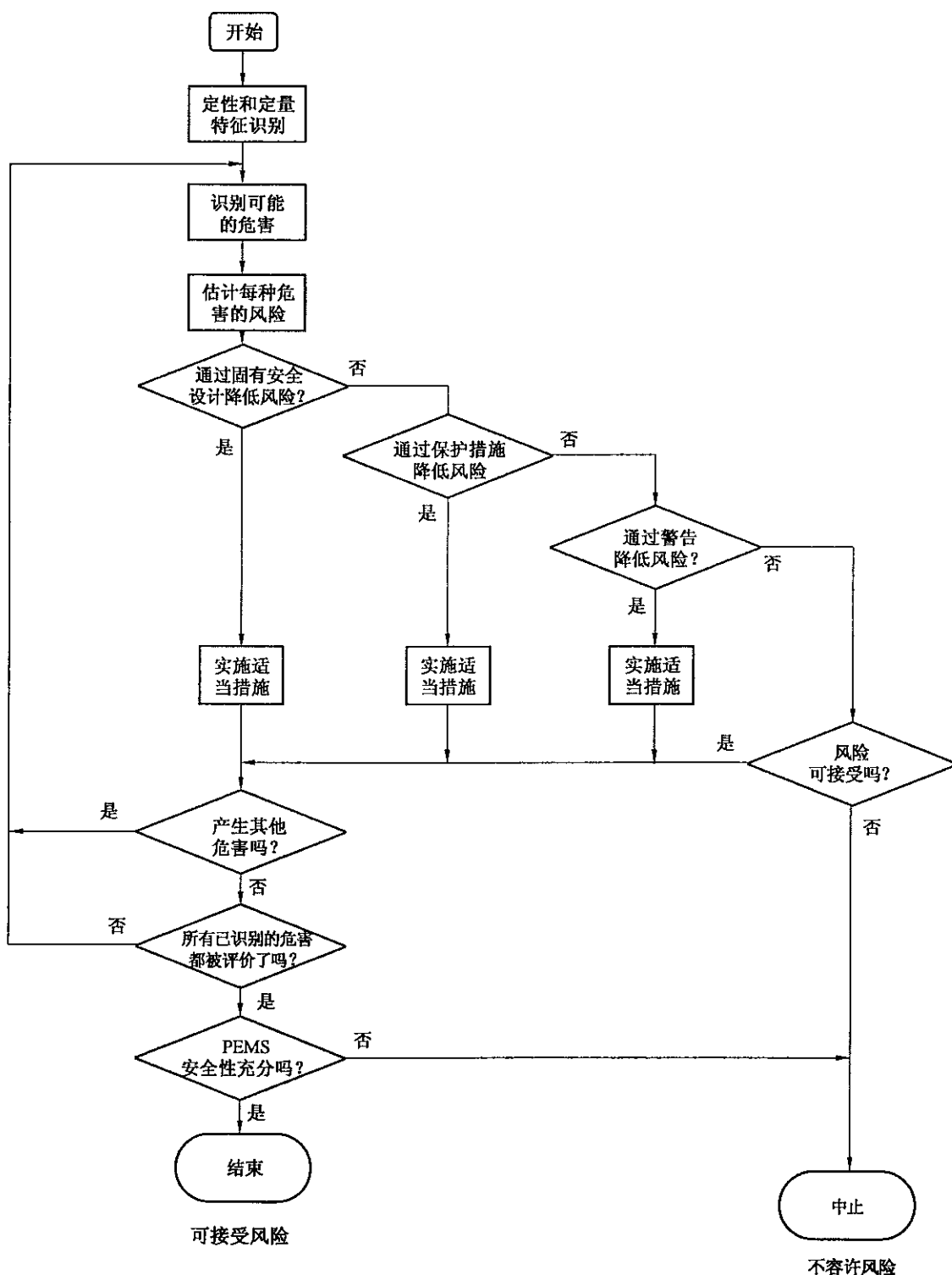
图 CCC. 2 风险管理过程
