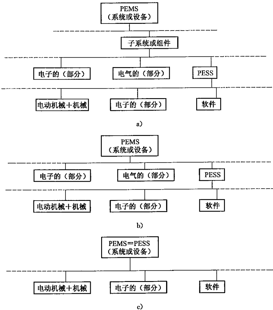
图 EEE.1 PEMS/PESS 体系结构例子
