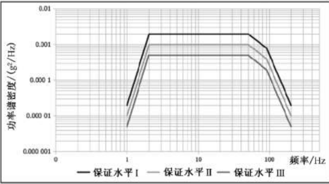
图 2 铁路试验的功率谱密度水平
