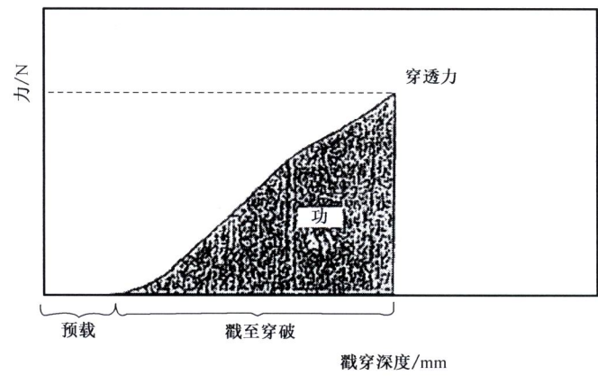
图 3 慢速戳穿试验图示输出
