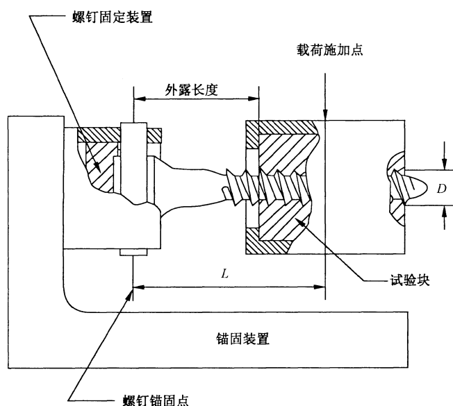
图 5 脊柱螺钉试验装置
