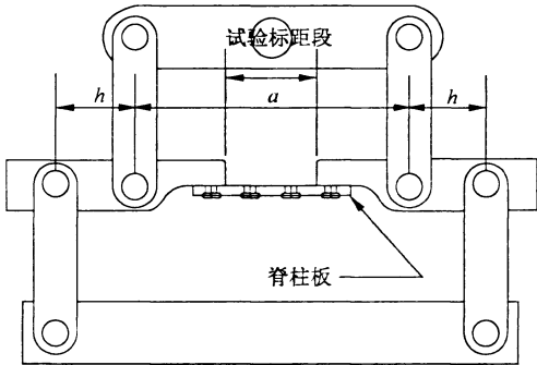
图 3 脊柱板试验装置, R = -1 加载
