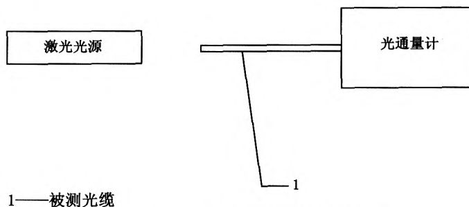
图 4 光能传递效率测量的试验装置
